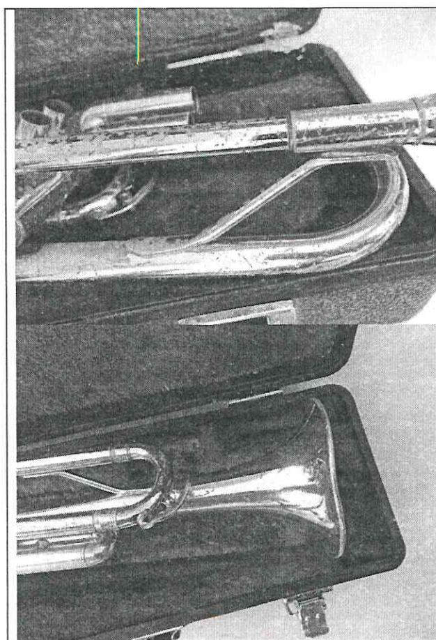
Diagnóstico del estado de los instrumentos, desmontaje de cada una de las partes y extracción de golpes en campana, cuerpo y bombas.
