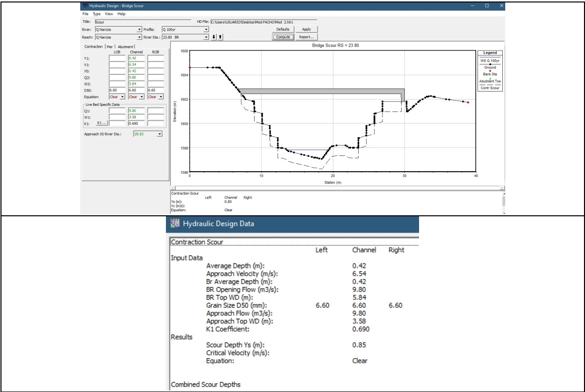
Imagen 42. Socavación en el puente calculado mediante el Hec Ras Fuente. Radicado CAR No. 08251002171 del 15 de diciembre de 2025- Municipio de Pacho
