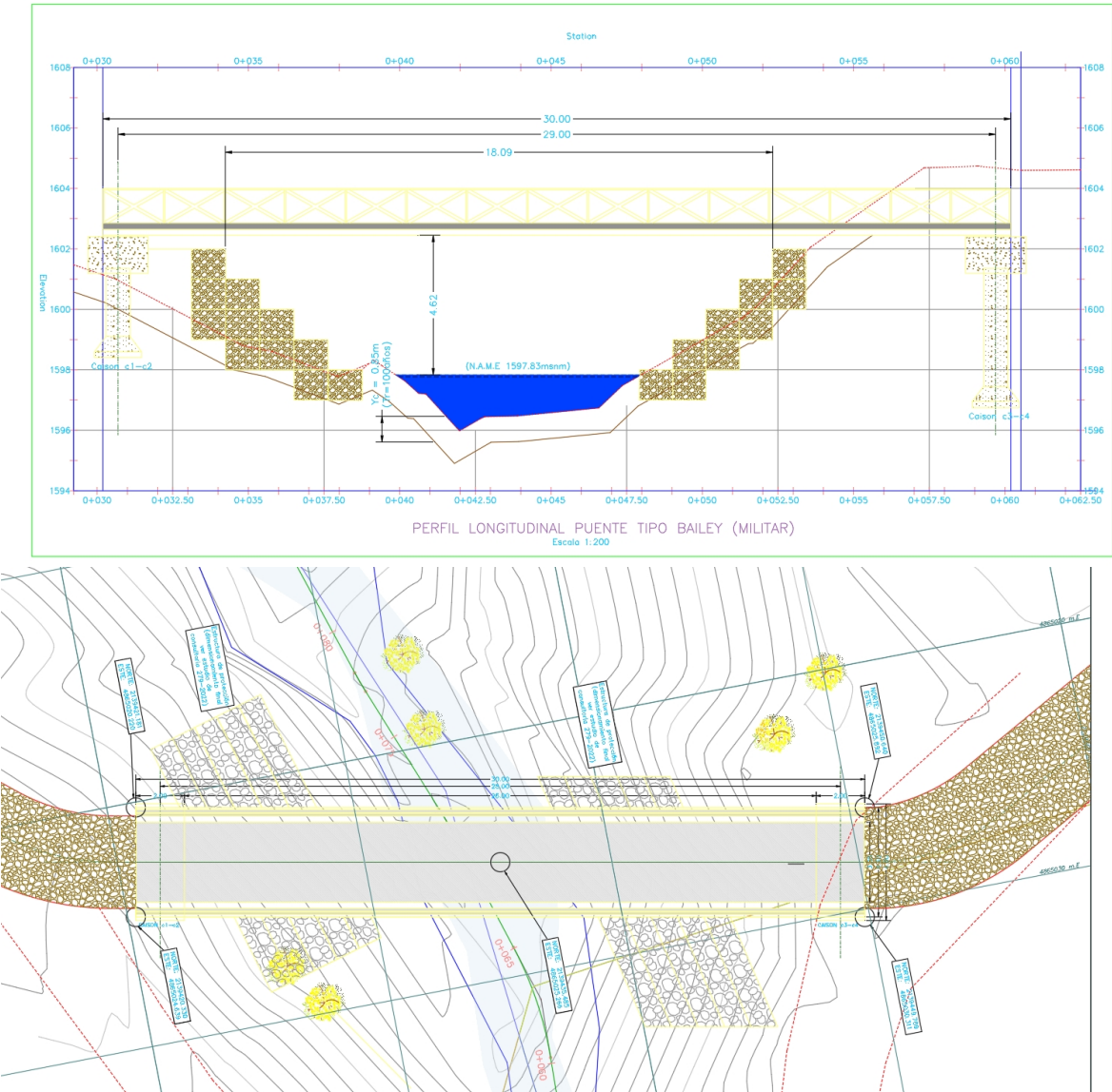
Imagen 11. Perfil Hidraulico Fuente. Radicado CAR No. 08251002171 del 15 de diciembre de 2025- Municipio de Pacho.
