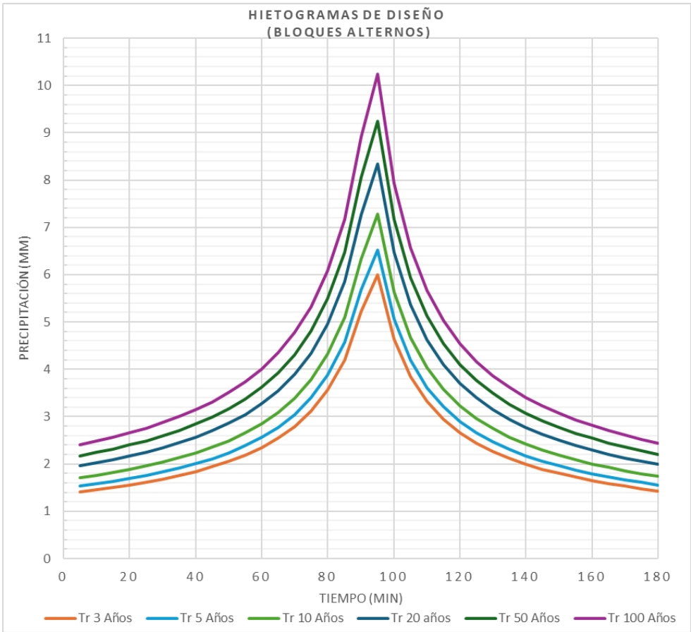
Imagen 27. Hietograma Fuente. Radicado CAR No. 08251002171 del 15 de diciembre de 2025- Municipio de Pacho.
