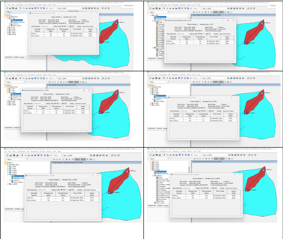
Imagen 31. Modelo HEC-HMS quebrada Narciza- Resultados Fuente . Radicado CAR No. 08251002171 del 15 de diciembre de 2025- Municipio de Pacho.
