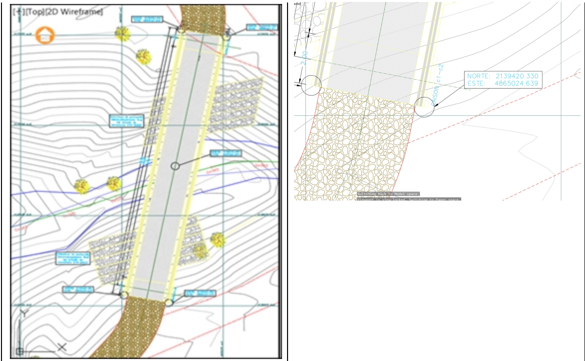
Imagen 10. Implantación de la Estructura Fuente. Radicado CAR No. 08251002171 del 15 de diciembre de 2025- Municipio de Pacho.
