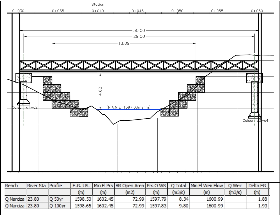
Imagen 39. Cota lamina de Agua 100 Años period de Retorno -HEC RAS Fuente. Radicado CAR No. 08251002171 del 15 de diciembre de 2025- Municipio de Pacho.
