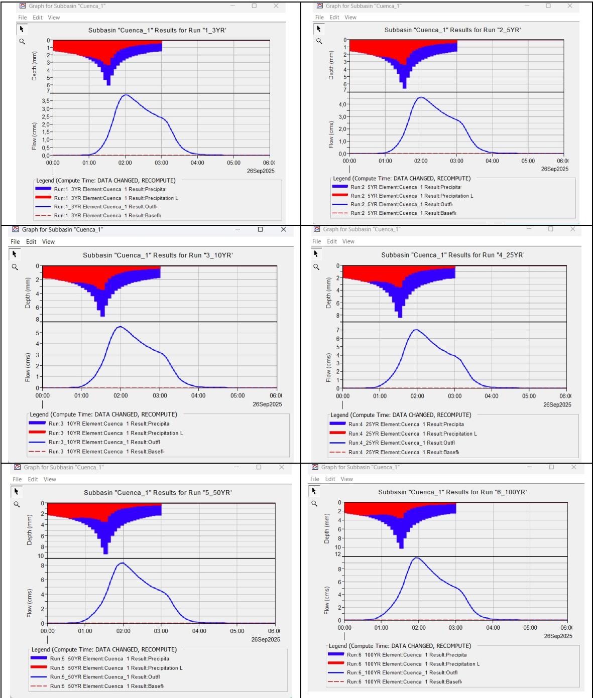
Imagen 30. Modelo HEC-HMS quebrada Narciza Fuente. Radicado CAR No. 08251002171 del 15 de diciembre de 2025- Municipio de Pacho.
