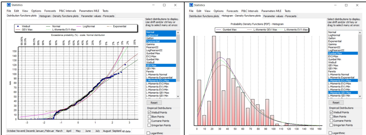
Imagen 23. Hydrognomon- Analisis Estadístico Fuente. Radicado CAR No. 08251002171 del 15 de diciembre de 2025- Municipio de Pacho.
