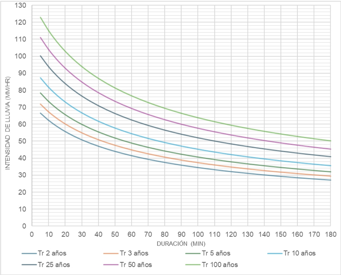
Imagen 25. Curvas IDF aplicando la distribución GEV-MAX - Hydrognomon Fuente. Radicado CAR No. 08251002171 del 15 de diciembre de 2025- Municipio de Pacho.
