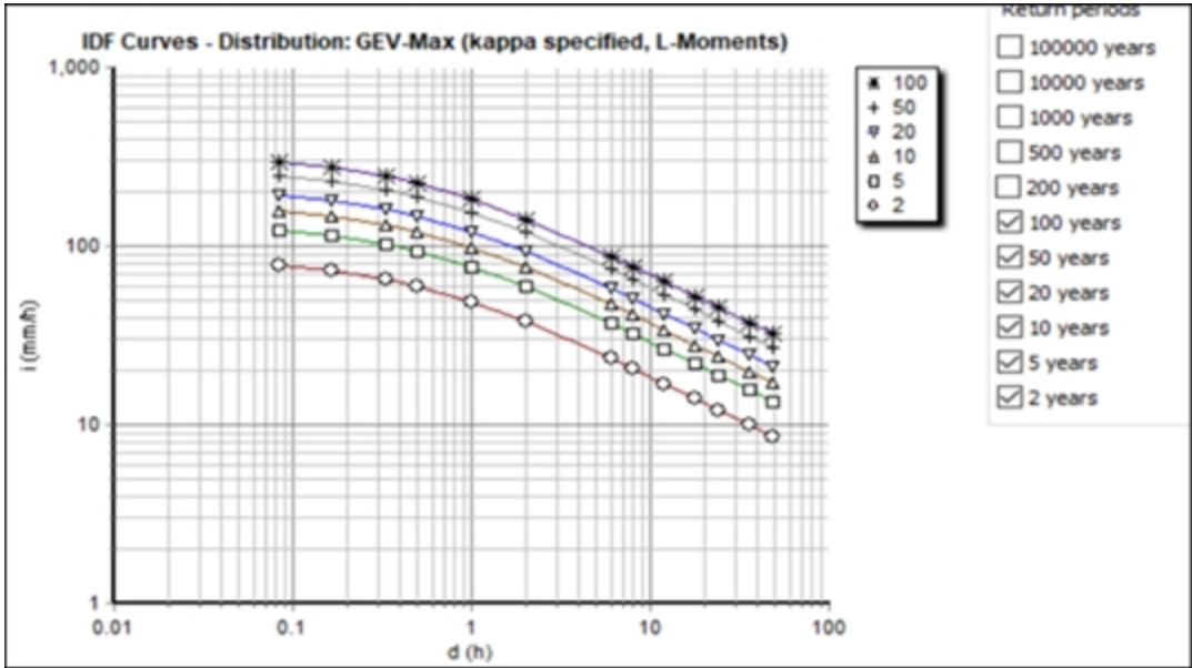
Imagen 25. Curvas IDF aplicando la distribución GEV-MAX - Hydrognomon Fuente. Radicado CAR No. 08251002171 del 15 de diciembre de 2025- Municipio de Pacho.
