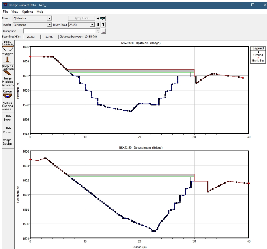
Imagen 36. Implantación - Bride data - HEC RAS Fuente. Radicado CAR No. 08251002171 del 15 de diciembre de 2025- Municipio de Pacho.
