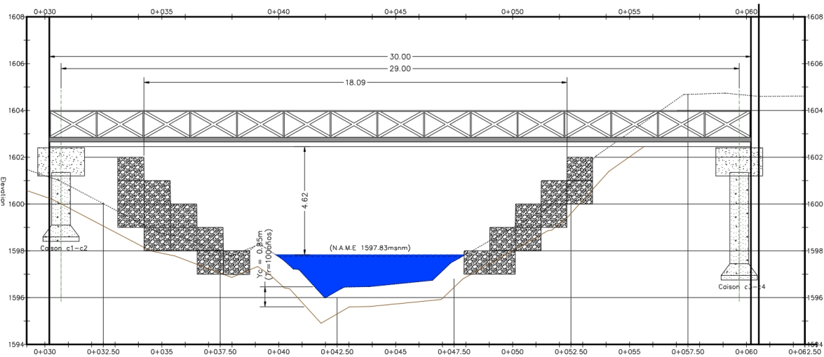
Imagen 43. Socavación en el puente calculado mediante el Hec Ras Fuente. Radicado CAR No. 08251002171 del 15 de diciembre de 2025- Municipio de Pacho
