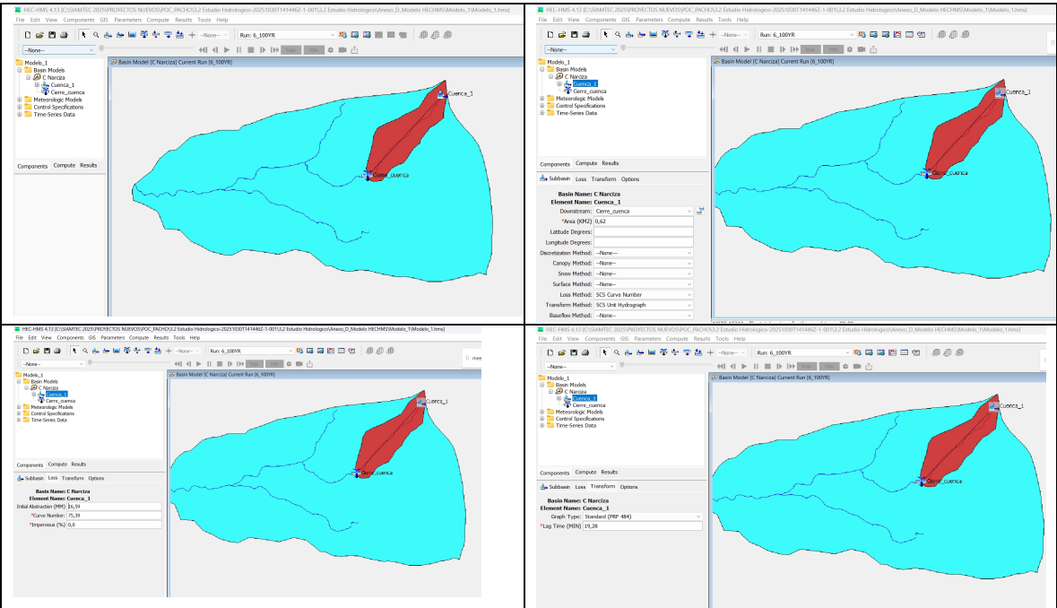
Imagen 29. Modelo HEC-HMS quebrada Narciza en el punto de cierre Parametrización Fuente. Radicado CAR No. 08251002171 del 15 de diciembre de 2025- Municipio de Pacho.
