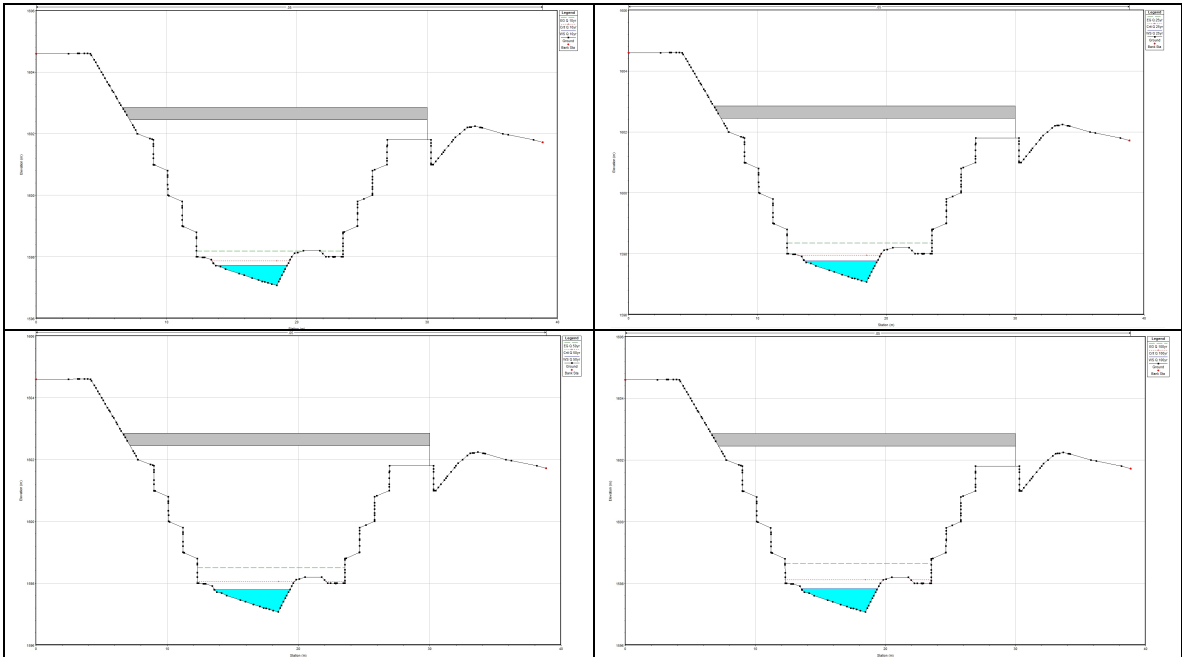
Imagen 38. Sección puente lámina de agua TR10, TR25, TR50 Y TR100 años -HEC RAS Fuente. Radicado CAR No. 08251002171 del 15 de diciembre de 2025- Municipio de Pacho.
