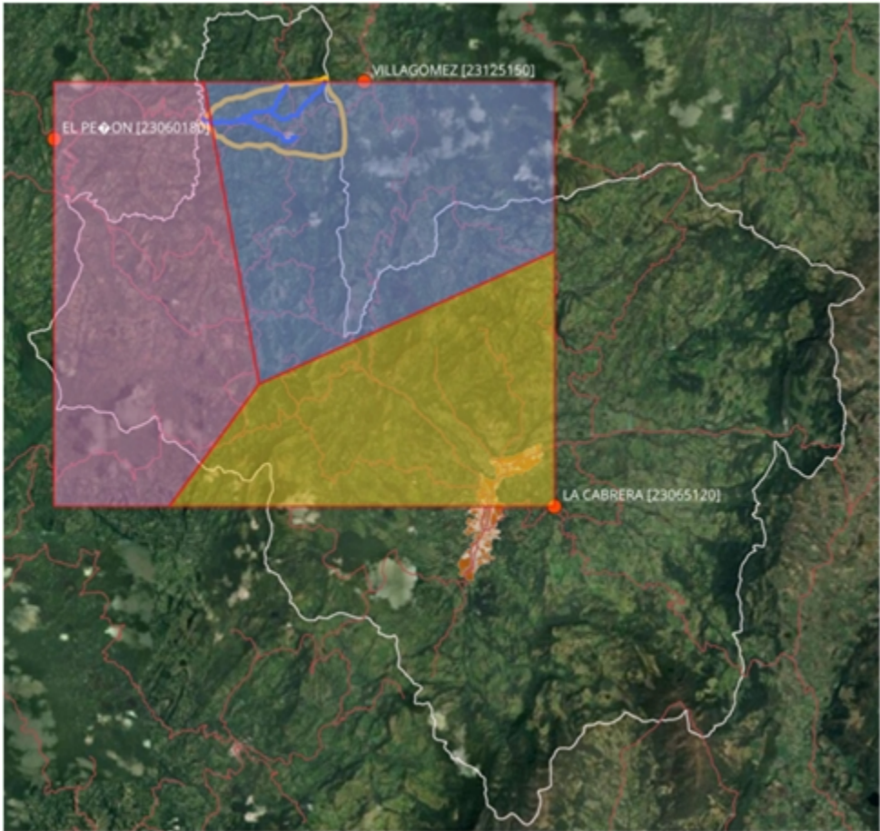
Imagen 22. Analisis de Poligonos de Thiessen Fuente. Radicado CAR No. 08251002171 del 15 de diciembre de 2025- Municipio de Pacho.
