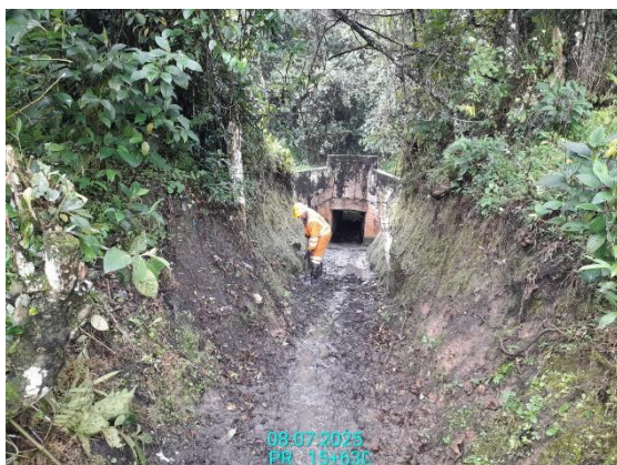
CARRETERA: BARBOSA-TUNJA (6209) SITIO: PR15+0630 DESCRIPCIÓN: LIMPIEZA DESCOLE OBRA DE DRENAJE FECHA: 08 de julio de 2025
