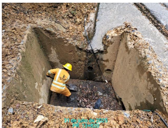
CARRETERA: BARBOSA-TUNJA (6209) SITIO: PR13+0820 DESCRIPCIÓN: LIMPIEZA OBRA DE DRENAJE FECHA: 31 de julio de 2025
