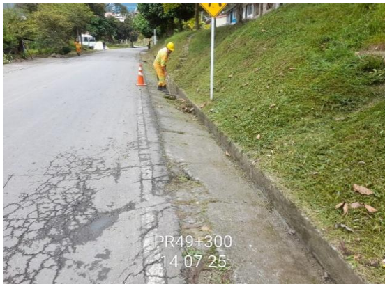
CARRETERA: OTANCHE - CHIQUINQUIRÁ (6007) SITIO: PR49+0300 DESCRIPCIÓN: LIMPIEZA DE CUNETAS FECHA: 14 de julio de 2025
