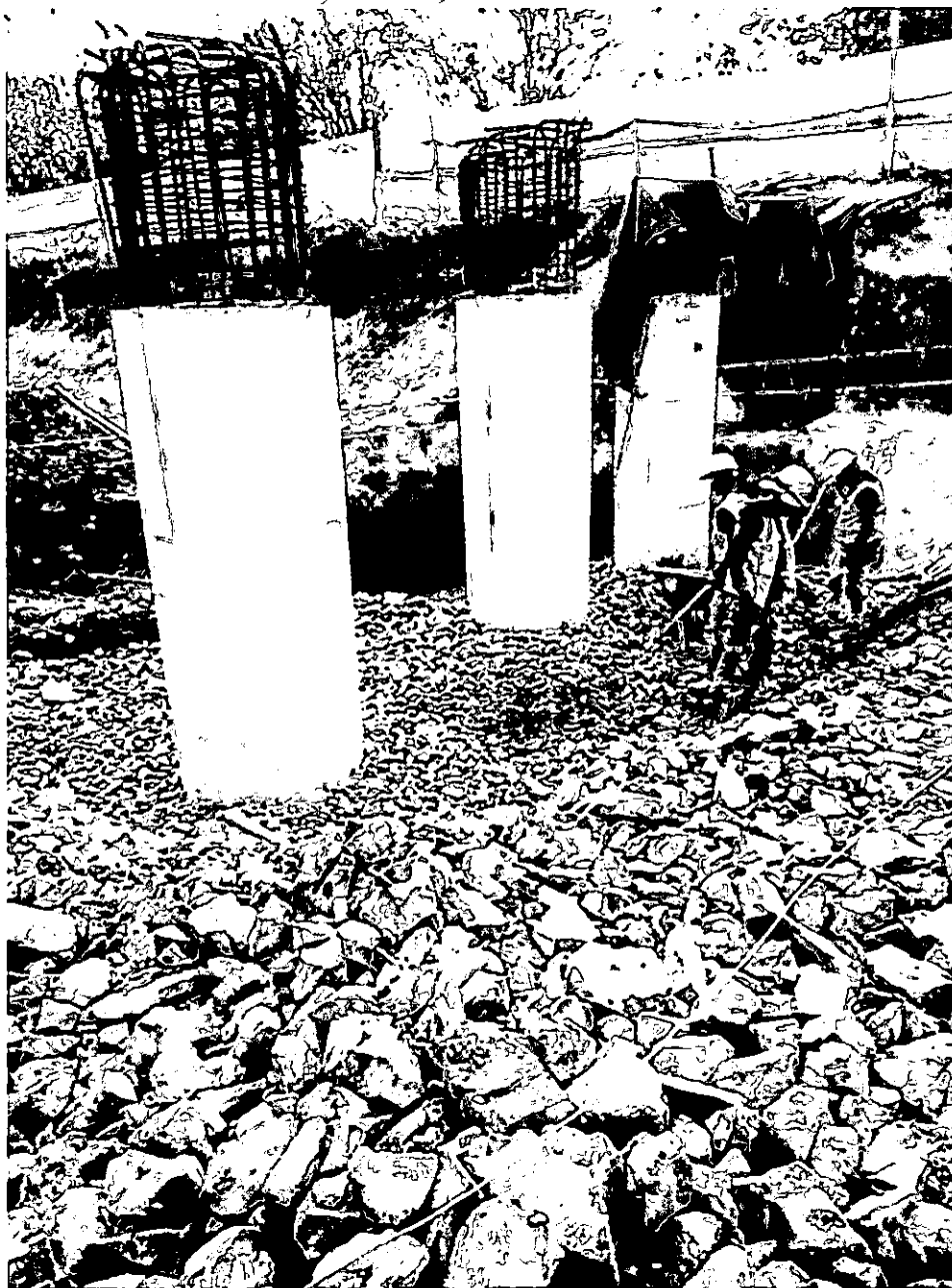
Imagen 11. Fundición de estructuras
