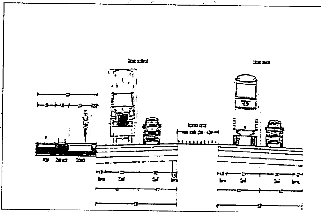
Imagen 3. Sección Transversal del proyecto. Fuente: Anexo Técnico No. 1 LP-SIV-001-2025).
