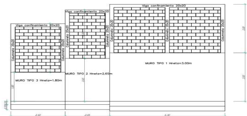
ALZADO MURO DE CERRAMIENTO EN MAMPOSTERÍA CONFINADA ESC. 1:50
