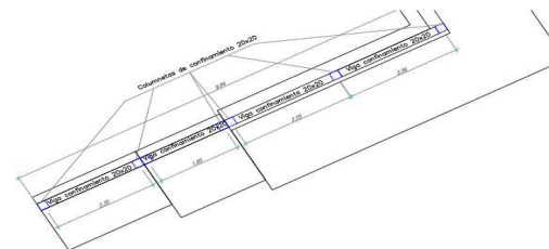
PLANTA MURO DE CERRAMIENTO EN MAMPOSTERÍA CONFINADA ESC. 1:50
