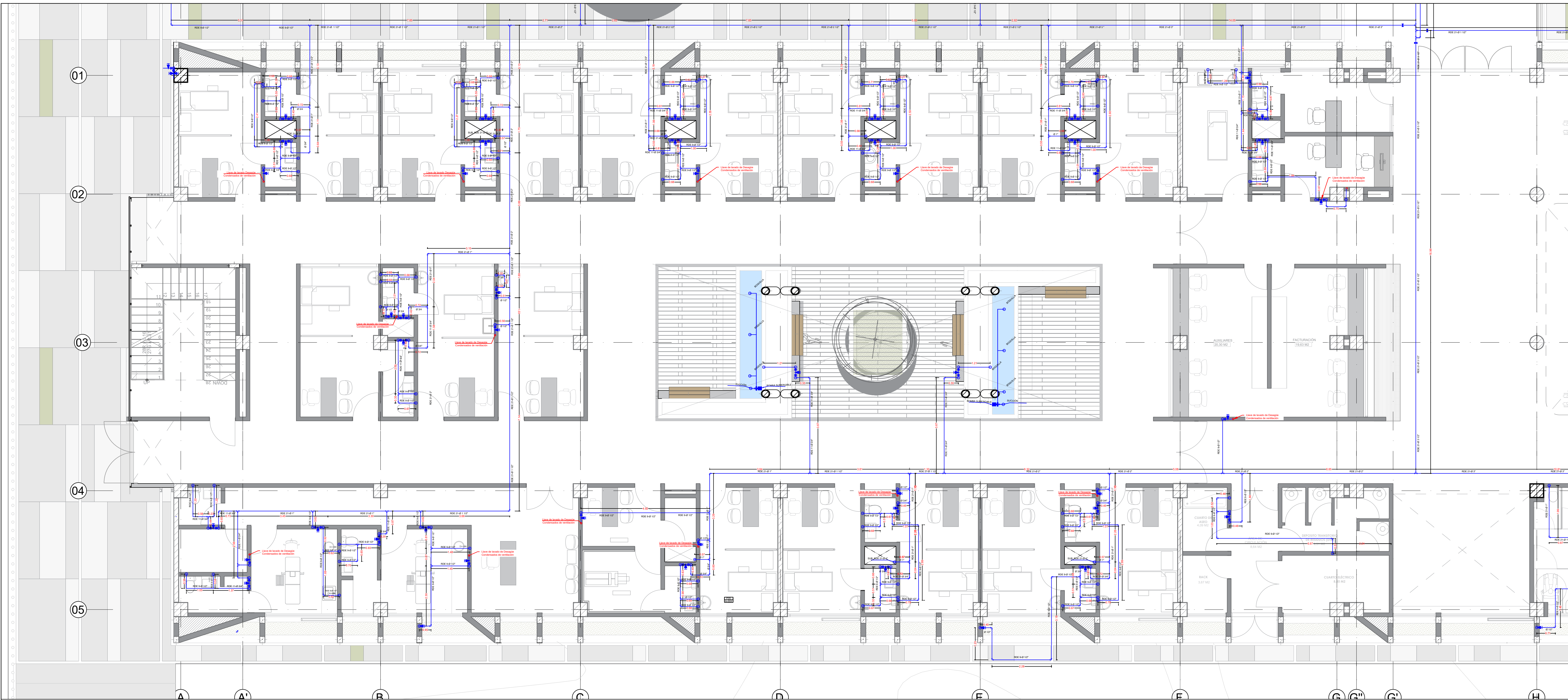
PLANTA PRIMER PISO INSTALACIONES HIDRÁULICAS
