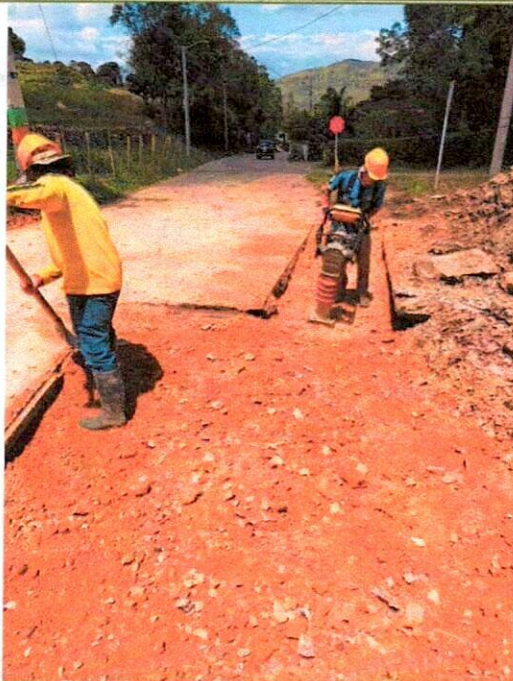
SUB BASE COMPACTADA (Imagen 1)
