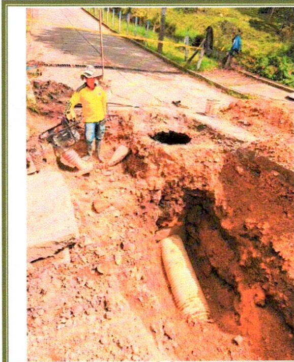
INSTALACIÓN DE TUBERÍA PVC 20" (imagen 1)
