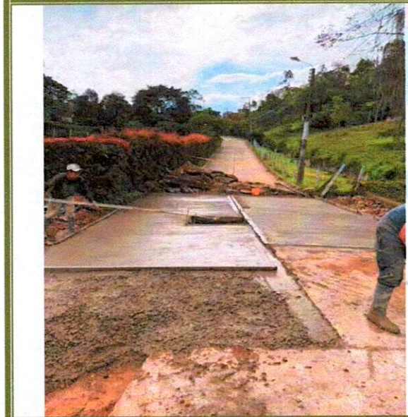
CONCRETO 3500 PSI
