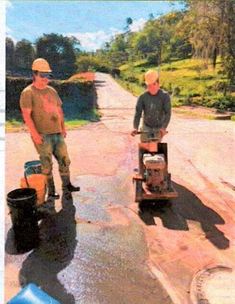
CORTE DE PAVIMENTO
