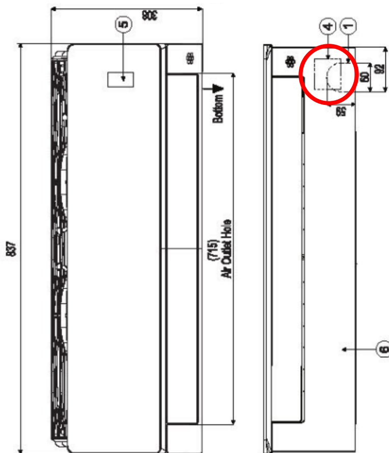
Imagen 2. Detalle aire acondicionado Mini Split 12000 BTU LG: (1) Bloque de terminales para suministro y comunicación (4) Acceso para refrigerante, desagüe y cableado eléctrico.
