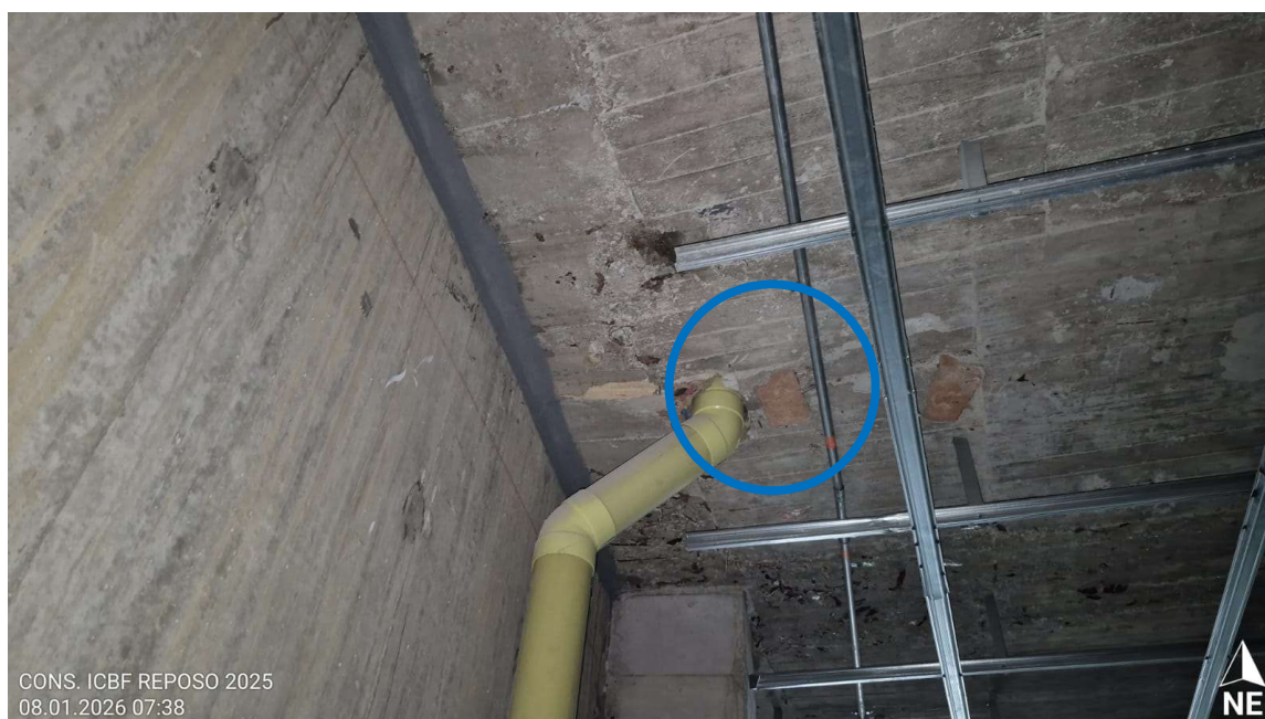
Imagen 1. Punto de filtración, gotera, en módulo de Nutricionista 02 en placa de techo en N0.00 – 4.00 m.
