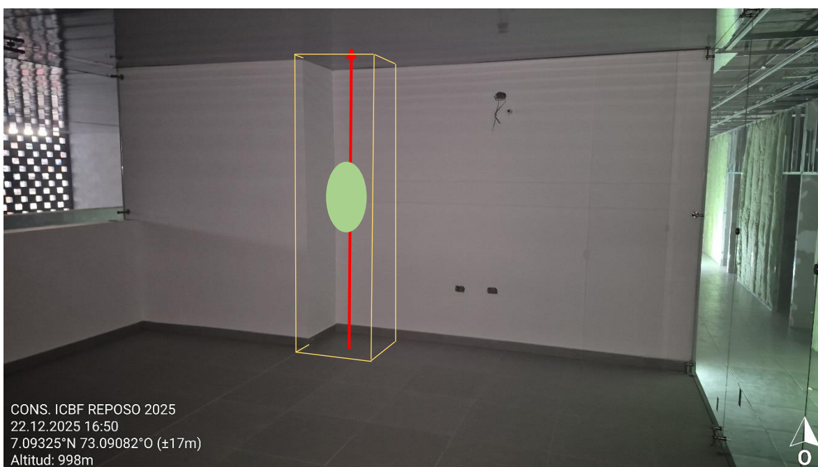
Imagen 8. Ludoteca N 0.00 – 4.00 m: Columna falsa (amarillo) para ocultar canalizaciones de ductos de comunicaciones y eléctricos (rojo). Se recomienda la implementación de ventana de inspección en caso de no hacer uso de tuberías para el cambio de nivel, medidas preliminares de 60x40 cm (alto – ancho).
