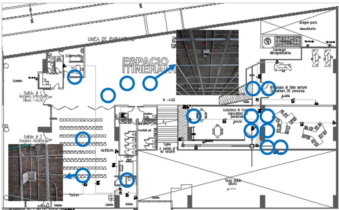
Imagen 2. Ubicación de cajas de inspección eléctricas con necesidad de ventana de inspección para realización de trabajos eléctricos.
