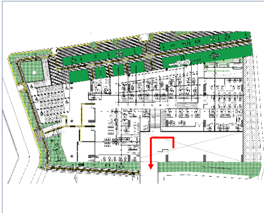
Imagen 2. Vista de planta trayecto original para paso de bandeja portacables y redes eléctricas complementarias. Longitud del trayecto original mayor.
