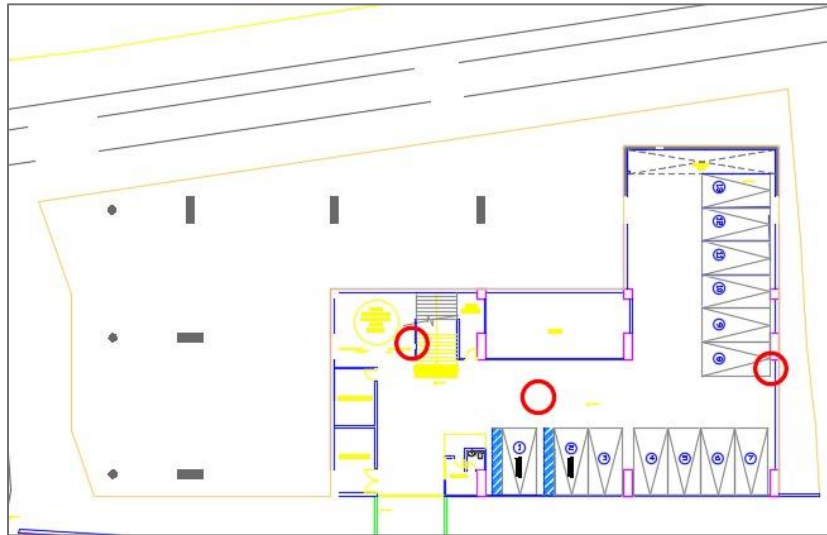
Figura 1. Resumen de filtraciones en zona de parqueadero N 0.00 -7-00 m
