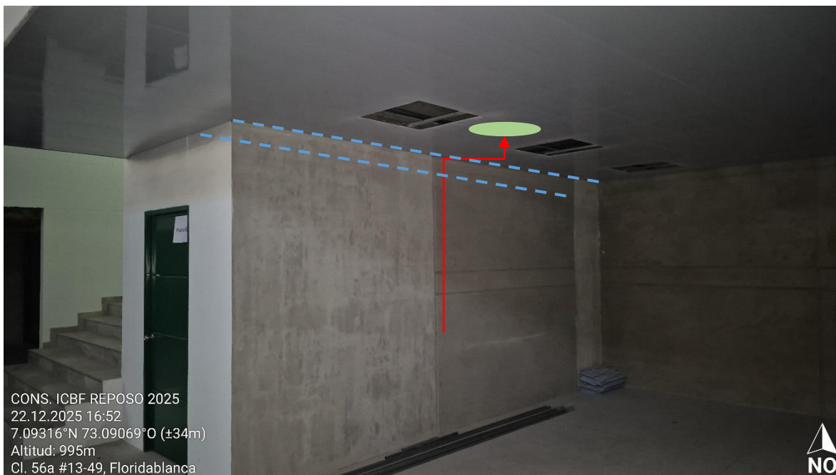
Imagen 7. Parqueadero N 0.00 – 7.00 m: Zona bajante del trayecto de ductos para red eléctrica y comunicaciones propuesta (rojo). Se debe desplazar la extracción del núcleo fuera del eje de la viga (azul) para cuidar su función estructural. Se propone ventana de inspección para futuros trabajos de mantenimiento.
