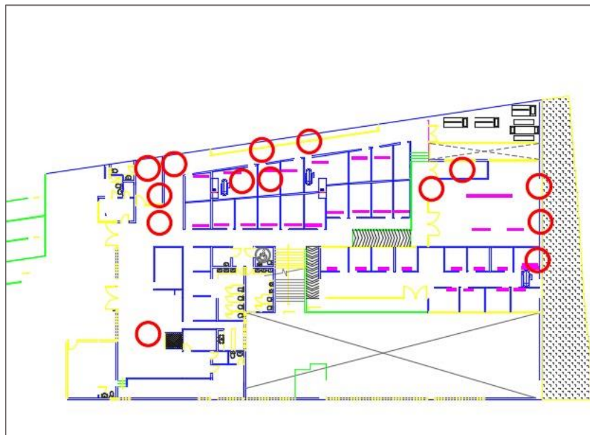
Figura 2. Resumen de filtraciones en zona de piso 1 N 0.00 -4-00 m
