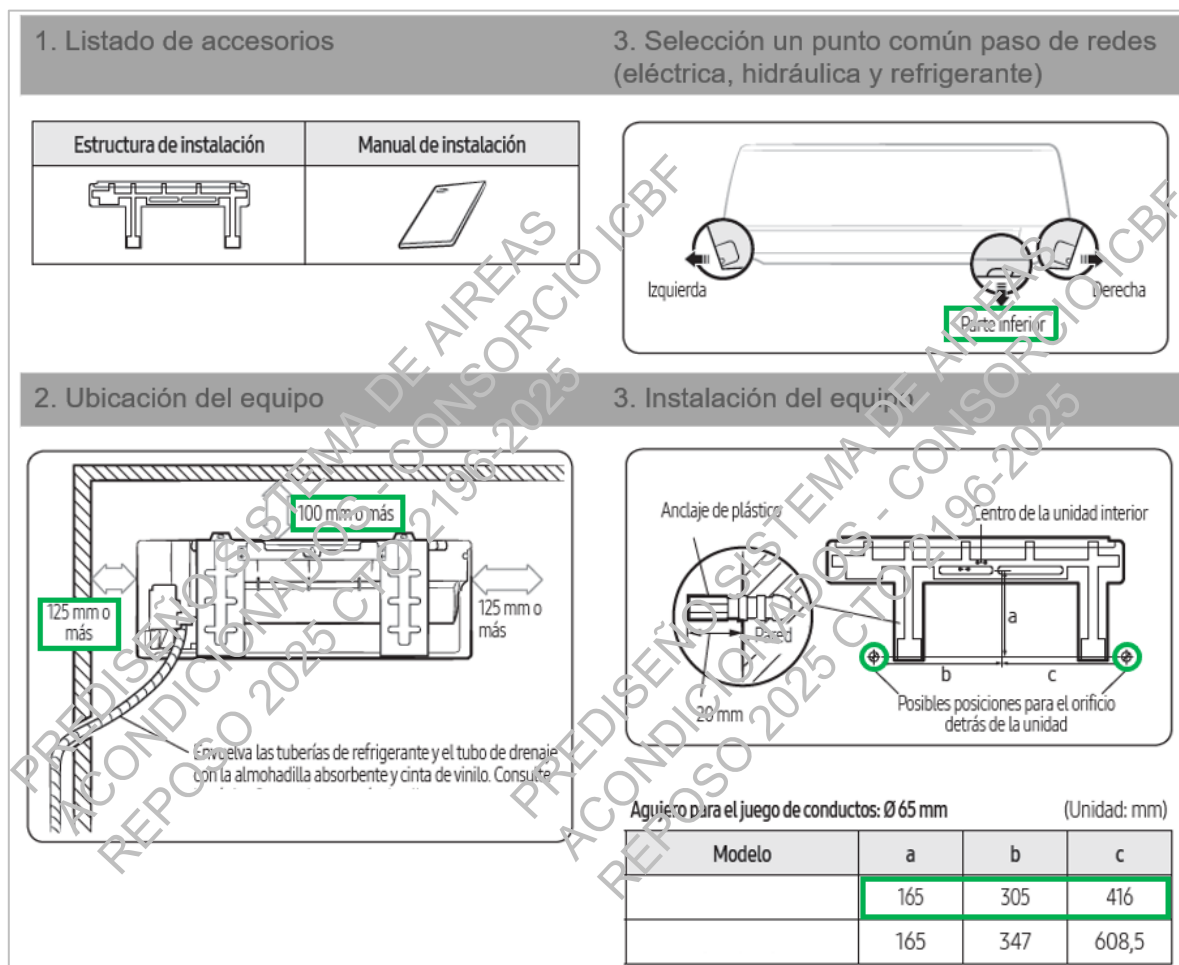
Figura 1. Especificaciones montaje y ubicación de salidas para unidad evaporadora en prediseño de sistema de aires acondicionados.
