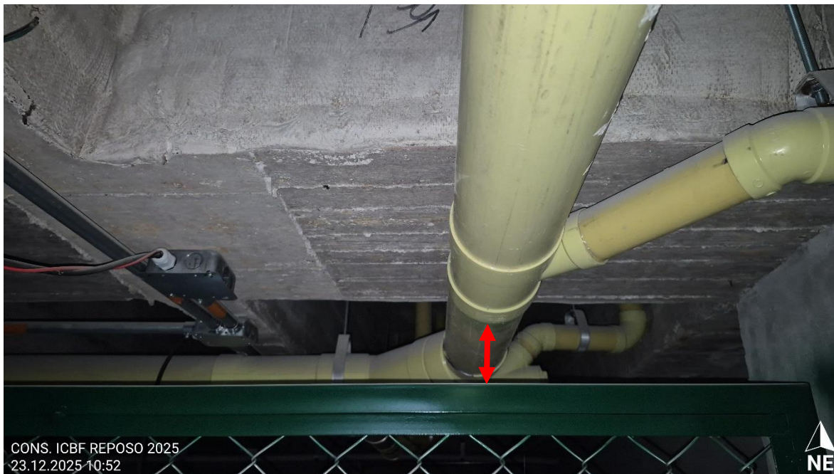
Imagen 4. Parqueadero N 0.00 – 7.00 m: Redes y ductos existentes en zona de parqueadero, cuarto de tanque. Se señala el espacio disponible para el paso de ductos y bandeja portacables.
