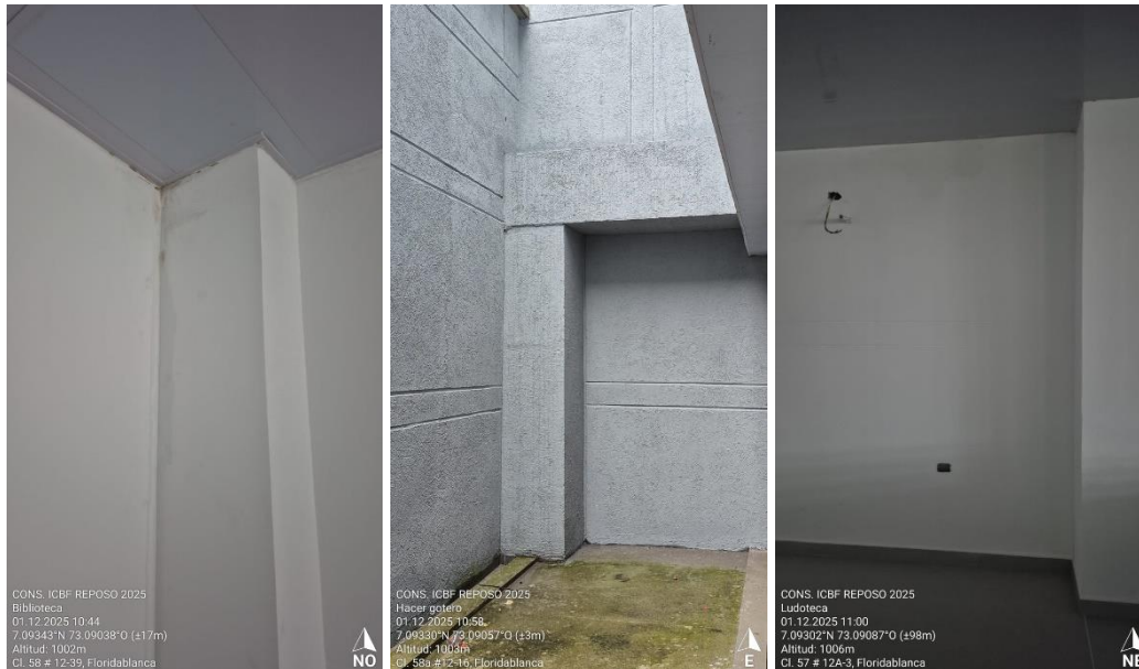
Imagen 2. Zonas de humedad presentadas acceso biblioteca, viga parqueadero, pantalla posterior ludoteca.
