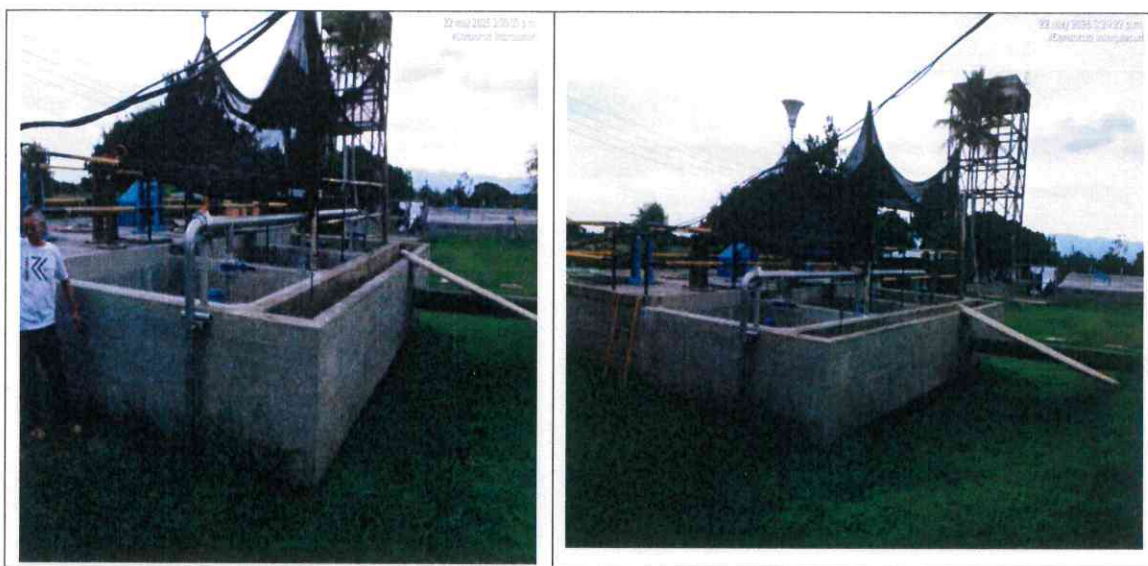
Suministro e Instalación de sopladores -Son dos unidades y en operación para las pruebas de los filtros
