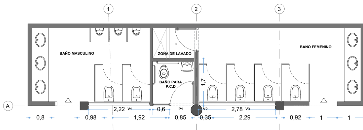
DISEÑO ARQUITECTÓNICO ACTUALIZADO BATERÍAS DE BAÑOS BLOQUE B
