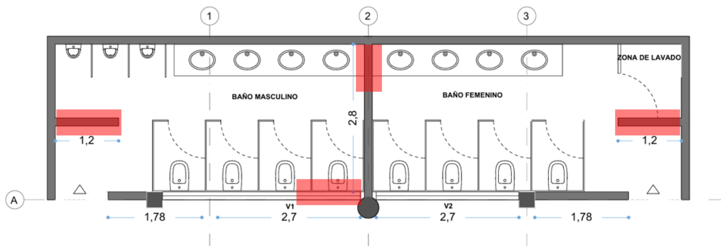
LEVANTAMIENTO ARQUITECTÓNICO/ ESTADO ACTUAL BATERÍAS DE BAÑOS BLOQUE B
