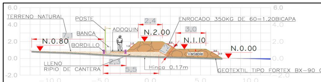
Figura 24. Sección tipo del enrocado longitudinal. Fuente: Elaborada por Aqua & Terra Consultores Asociados S.A.S, 2023.
