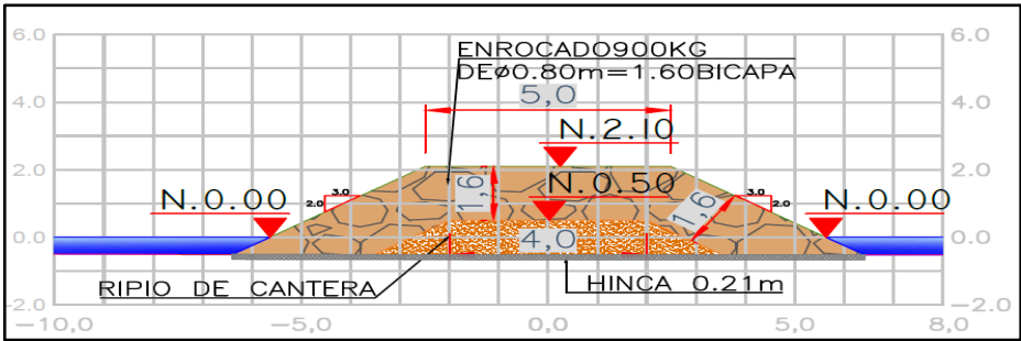
Figura 18. Sección tipo del cuerpo de la estructura del espolón. Fuente: Aqua & Terra Consultores asociados S.A.S, 2023.
