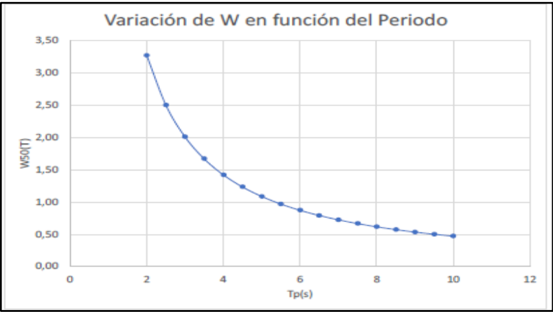
Figura 29. Variación del peso W en función del periodo medio Tp. Fuente: Elaborada por Aqua & Terra Consultores asociados S.A.S, 2022.
