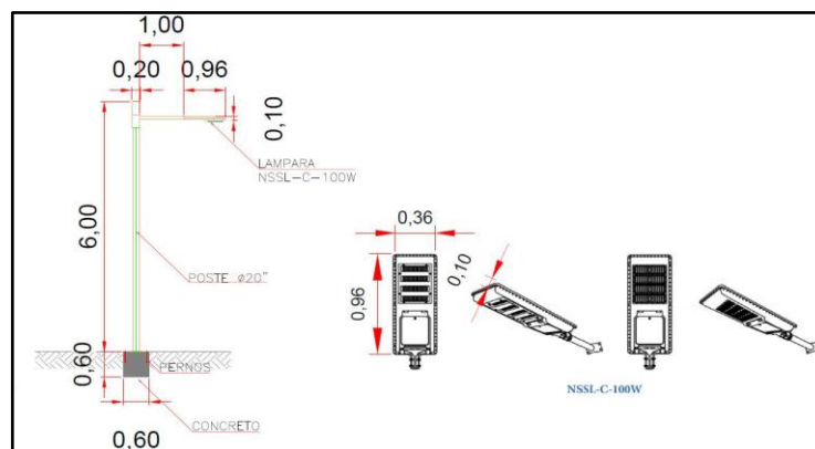
Figura 26. Luminaria en acero para urbanismo de Paseo Marítimo. Fuente: Aqua & Terra Consultores asociados S.A.S, 2023.
