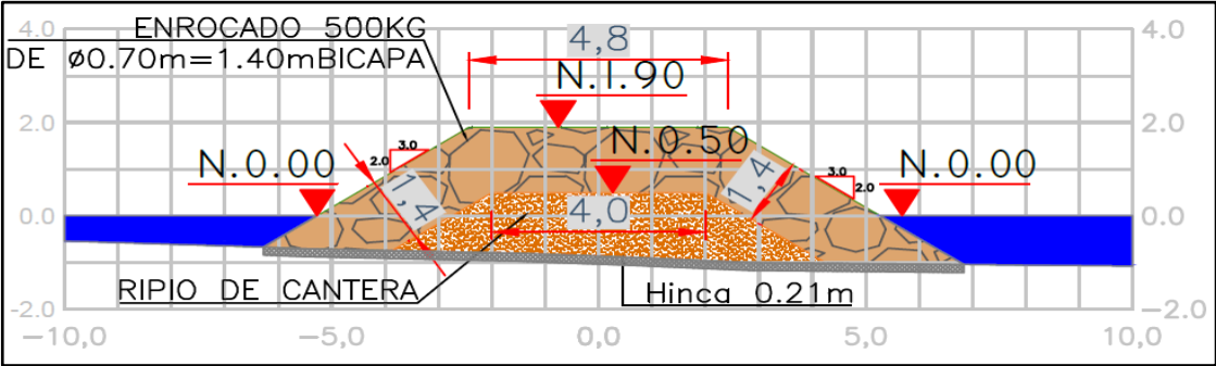
Figura 21. Sección tipo del cuerpo de la estructura del Tómbolo. Fuente: Aqua & Terra Consultores asociados S.A.S, 2023.
