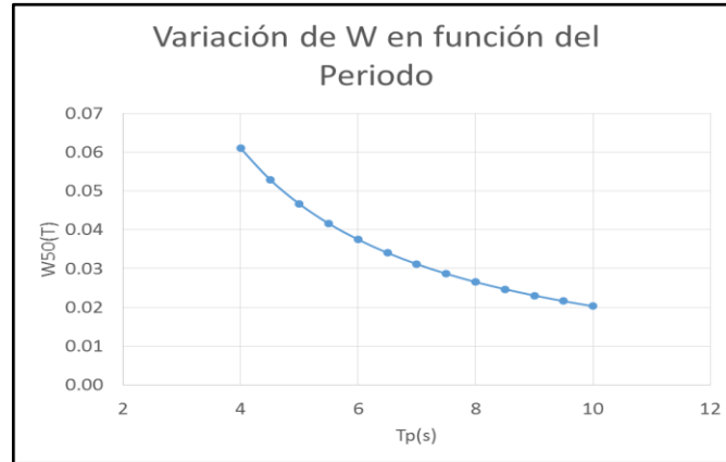
Figura 23. Variación del peso W en función del periodo medio Tp. Fuente: Elaborada por Aqua & Terra Consultores Asociados S.A.S, 2023
