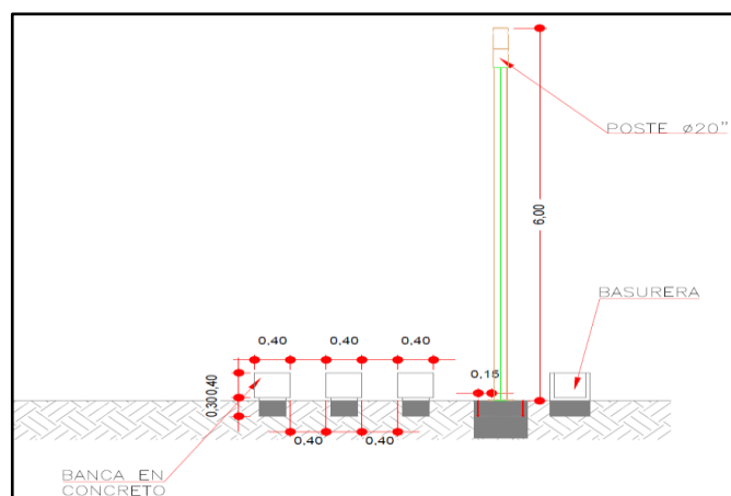
Figura 25. Sección longitudinal urbanismo de Paseo Marítimo Fuente: Aqua & Terra Consultores asociados S.A.S, 2023
