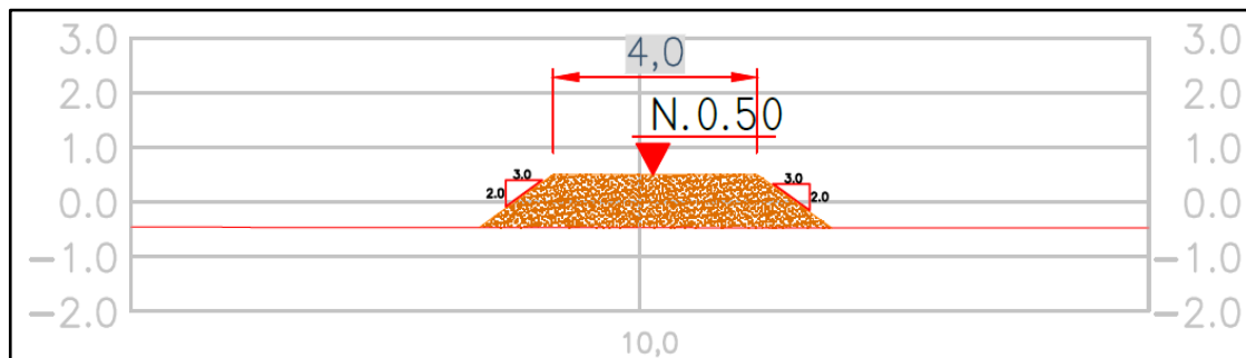
Figura 19. Sección tipo del vial de acceso a los tómbolos.
