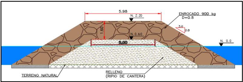
Figura 30. Sección tipo del cuerpo de la estructura del espolón. Fuente: Elaborada por Aqua & Terra Consultores Asociados S.A.S, 2022.
