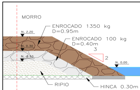
Figura 31. Sección tipo del morro.
