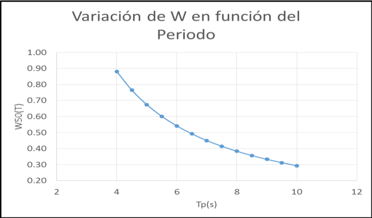
Figura 20. Variación del peso W en función del periodo medio Tp. Fuente: Aqua & Terra Consultores asociados S.A.S, 2023.
