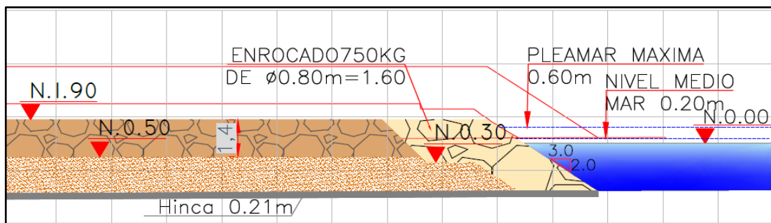
Figura 22. Sección tipo del morro del Tómbolo. Fuente: Aqua & Terra Consultores asociados S.A.S, 2023.
