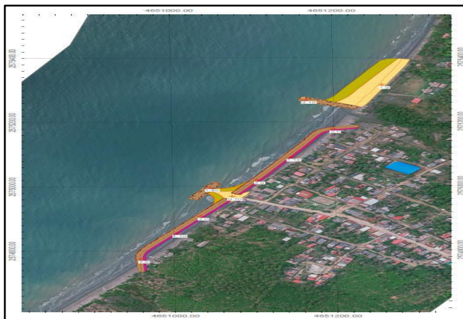
Figura 16. Planta Alternativa seleccionada para la zona de estudio. Fuente: Elaborado por Aqua & Terra Consultores Asociados S.A.S., 2023.
