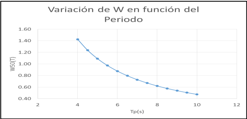
Figura 17. Variación del peso W en función del periodo medio Tp. Fuente: Aqua & Terra Consultores asociados S.A.S, 2023
