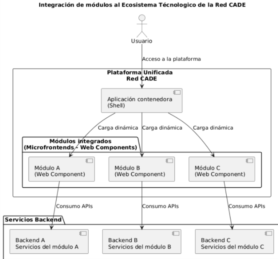
Imagen 3. Modelo de integración de módulos mediante microfrontends
