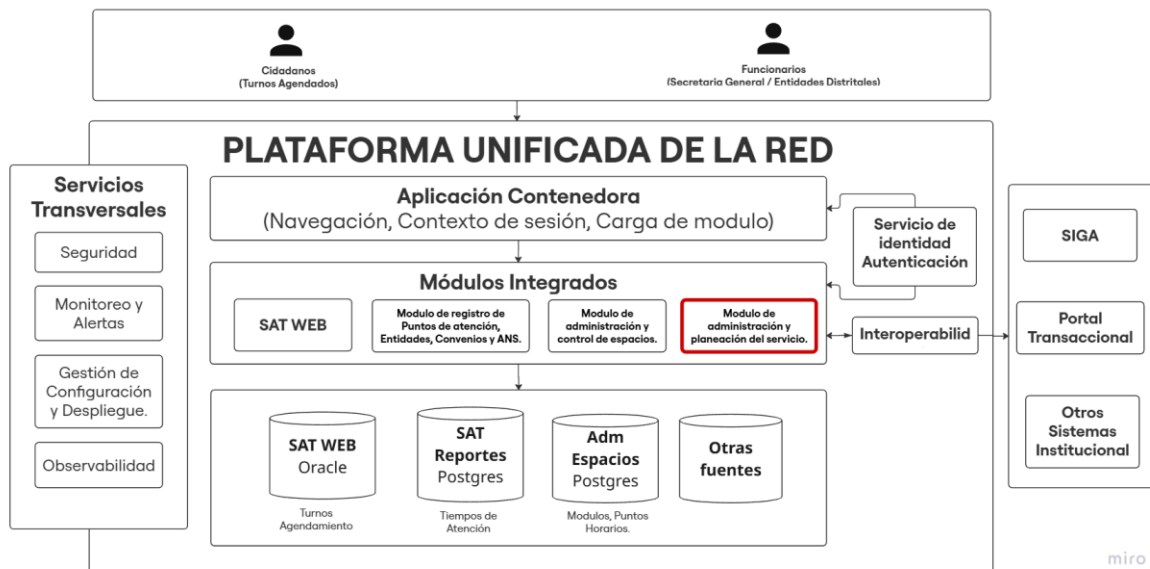
Imagen 2. Arquitectura conceptual de la Plataforma Unificada de servicios de la Red CADE
