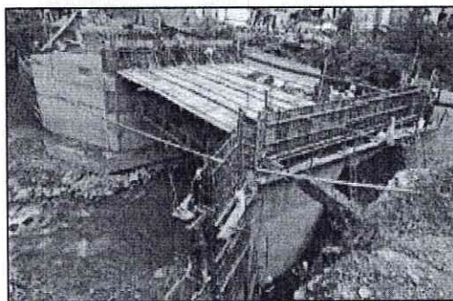
Anexo fotográfico 9. Manejo del caudal caño parrado MARGEN IZQUIERDA Y DERECHA CAÑO PARRADO
