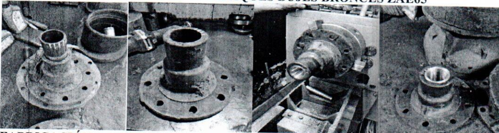
FABRICACIÓN Y CAMBIO DE 10 BUJES PARA CARCASA DE IMPULSORES EN BRONCE SAE65 DE 90MM X 58MM X 1 3/4"
