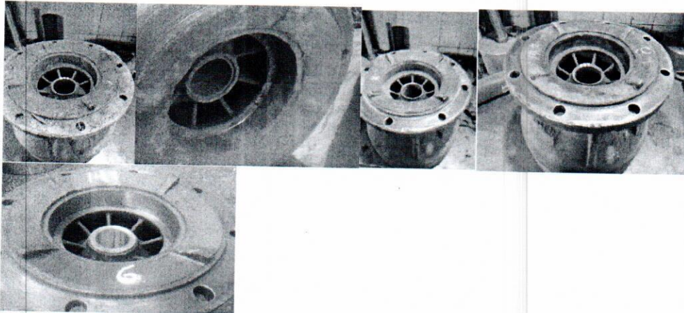
ENCAMISADA DE 10 IMPULSORES Y SOLDADA CON ANILLO EN BRONCE SAE65 DE 134MM X 148MM X 35MM
