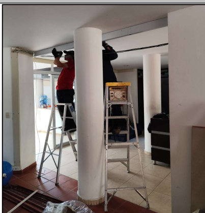
INSTALACIÓN ELECTRICA A 220V EN CANALETA METALICA
