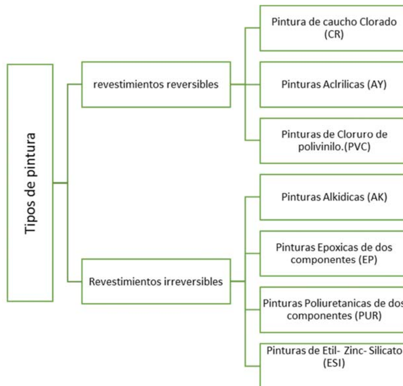
Figura 1. Clasificación de pinturas según sus aglutinantes
