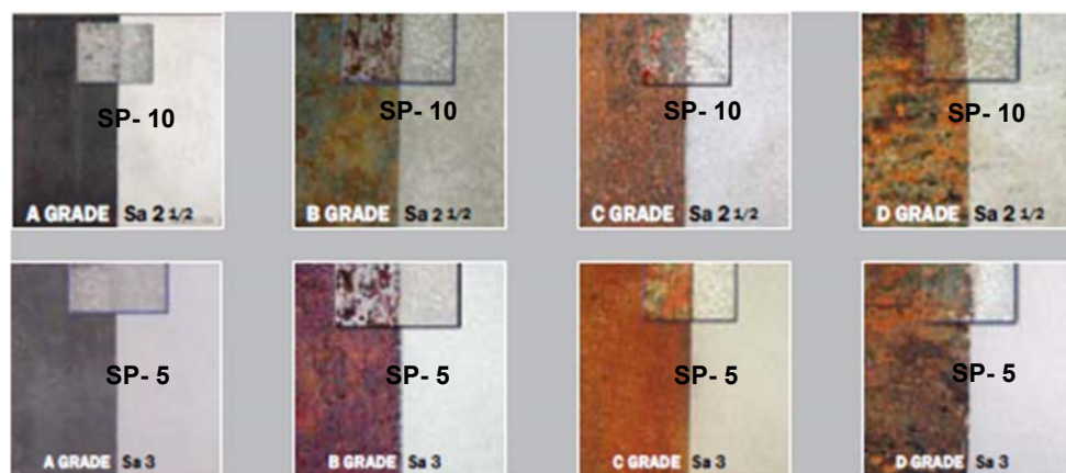
Ilustración 1. Grados de Oxidación y Grado de Limpieza aplicado: Tomado de SIKa, 2015.
