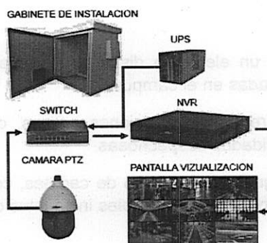
Topología general de conexión cámaras PTZ
