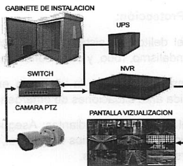
Topología general de conexión cámaras fijas/tipo bala/domo
