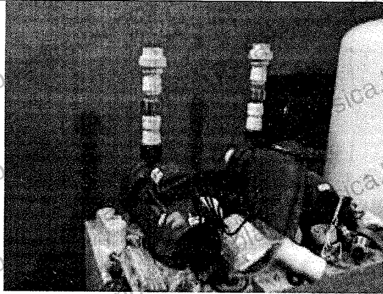
INSTALACION DEL SISTEMA AGUA POTABLE VARIADOR POR BOMBA 2 BOMBAS DE 10HP 220V TRIFASICO
