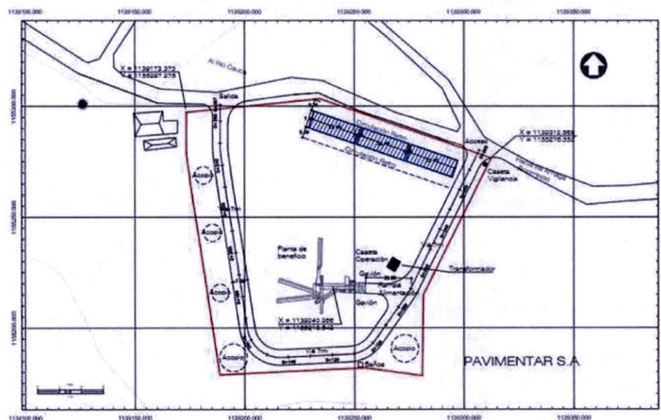
Figura 2. Esquema de las instalaciones adicionales propuestas, tomado de EIA Procopal S.A. 2019.
