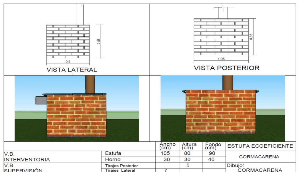
Figura 19 Diseño vista lateral y posterior. FUENTE: CORMACARENA 2025
