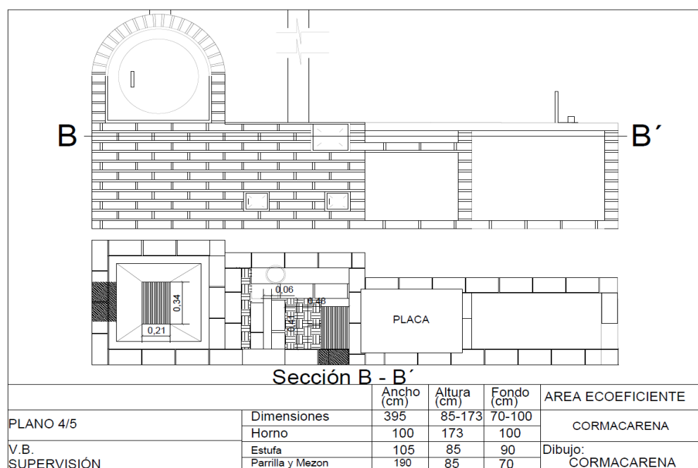
Figura 15 Diseño Sección B-B'. FUENTE: CORMACARENA
