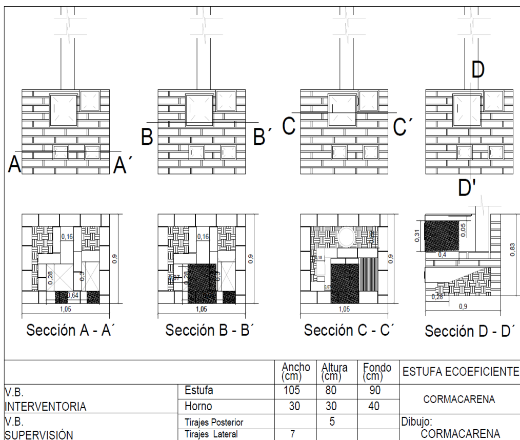
Figura 20 Diseño por secciones. FUENTE: CORMACARENA 2025
