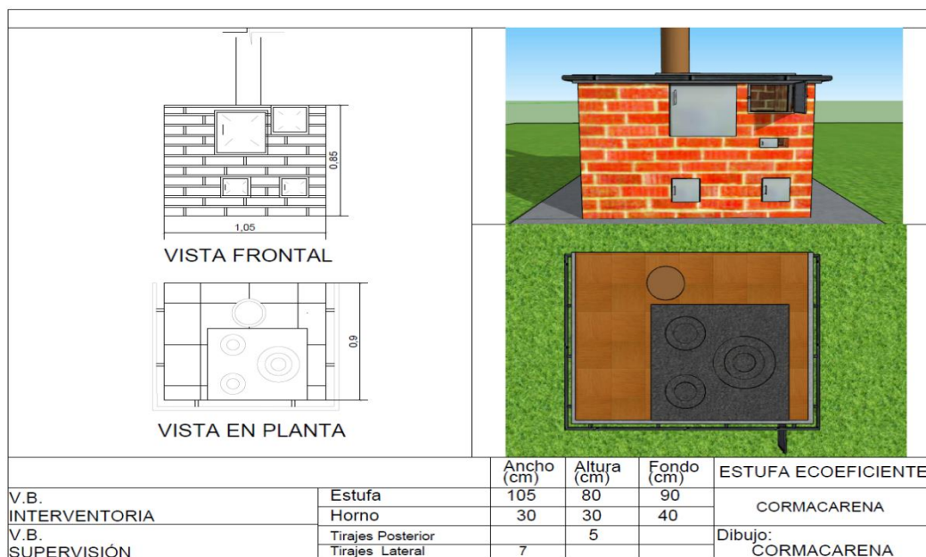
Figura 18 Diseño Vista frontal y en planta. FUENTE: CORMACARENA 2025
