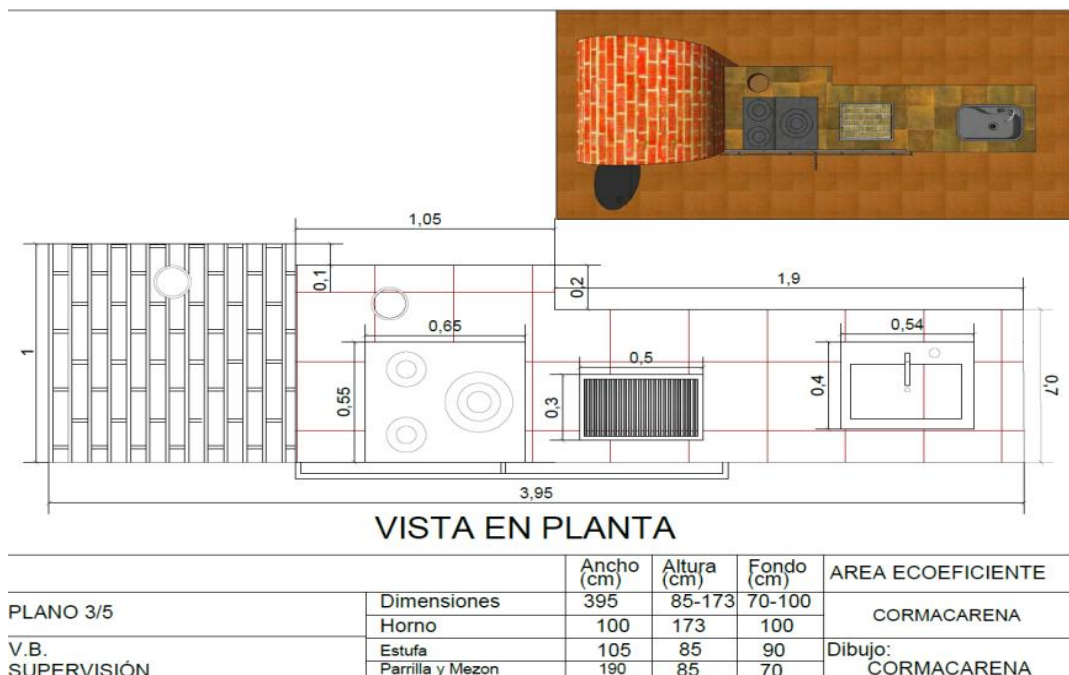
Figura 14 Diseño vista en planta. FUENTE: CORMACARENA 2025
