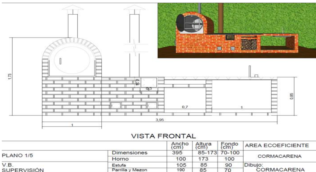
Figura 12 Diseño Vista frontal. FUENTE: CORMACARENA 2025.
