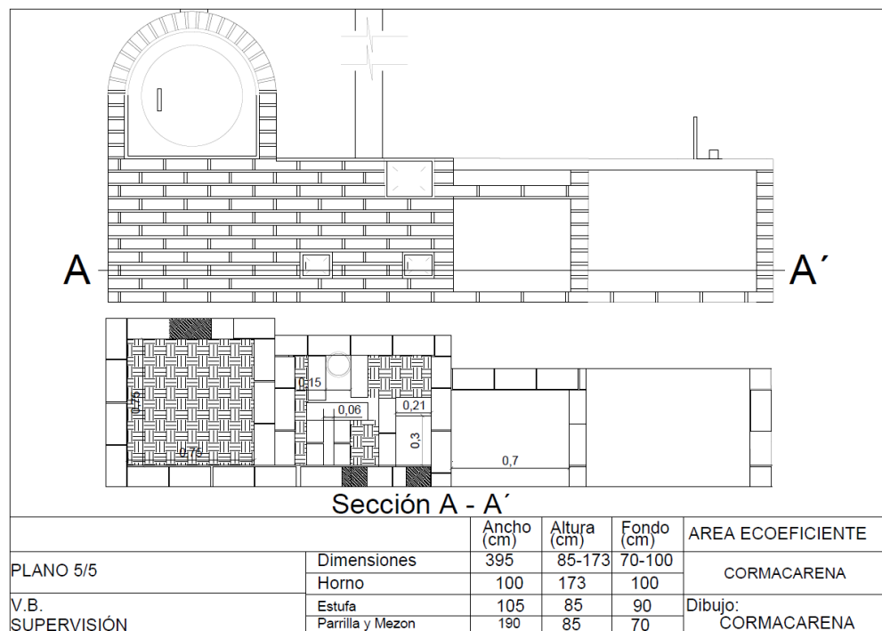
Figura 16 Diseño Sección A-A'. FUENTE: CORMACARENA 2025
