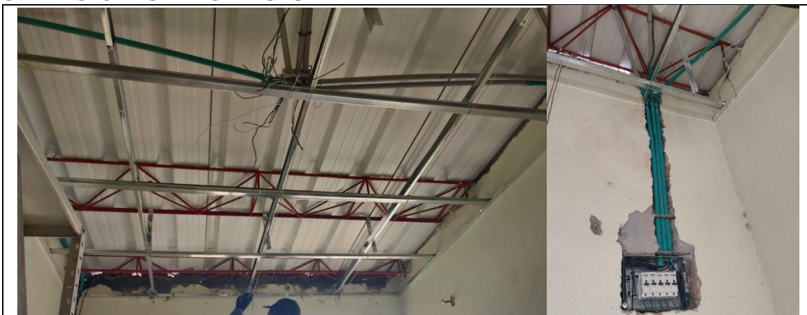
• Ilustración 6 – INSTALACIÓN DE TUBERIA ELECTRICA
