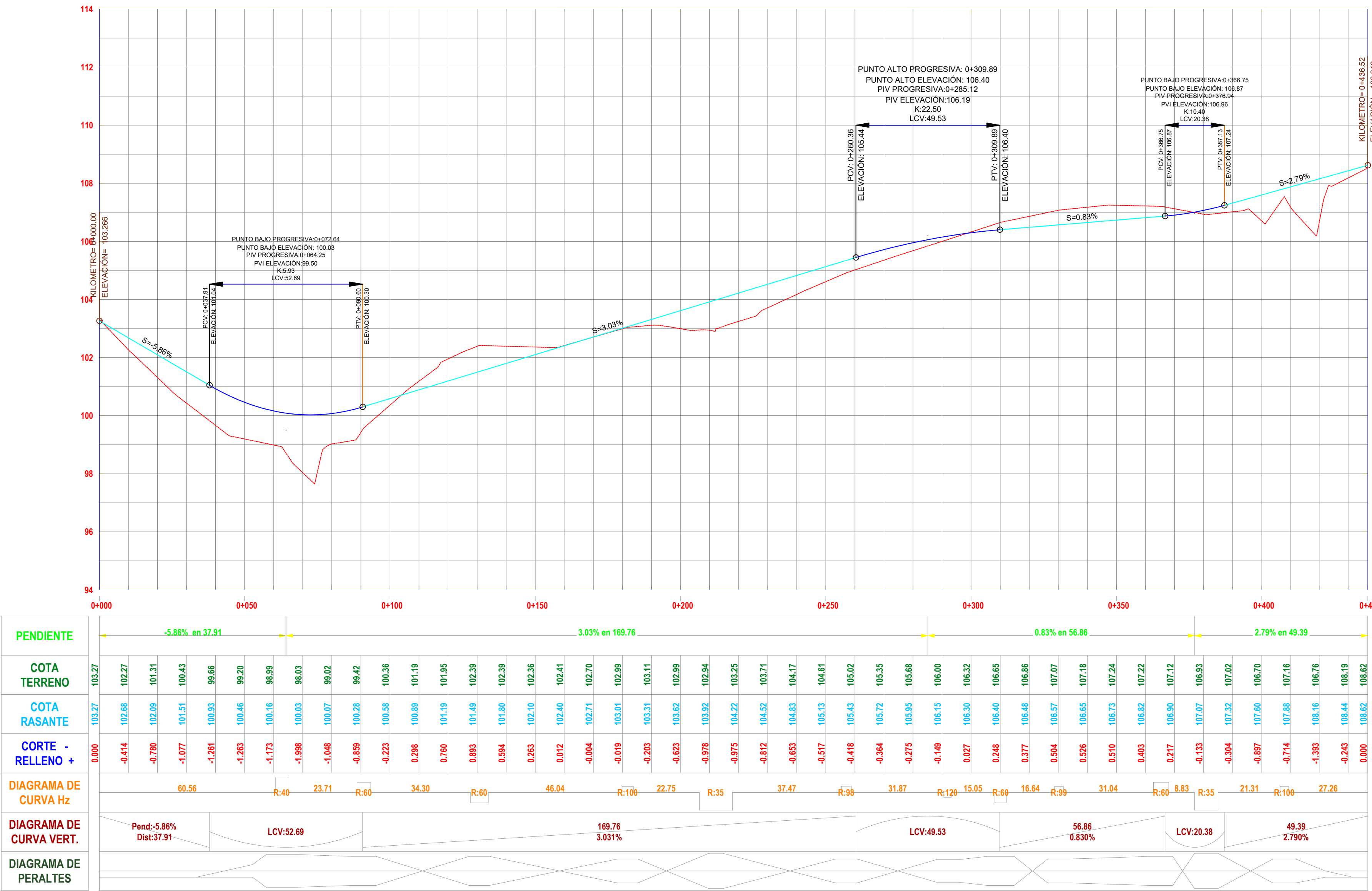
PERFIL LONGITUDINAL ESC.H = 1:1000 ESC.V = 1:100
