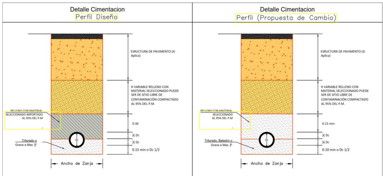
Ilustración 3. Perfiles aprobados por la interventoría para los llenos del Tramo 3 (desde la CADICA hasta la planta Guacarí)
