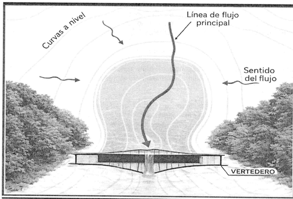
Figura 4. Esquema de reservorio sobre una línea de flujo natural
