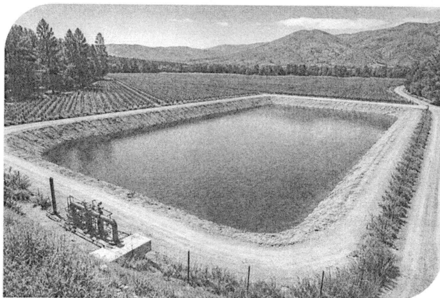
Foto No. 2: Imagen reservorio excavado para almacenamiento de agua
