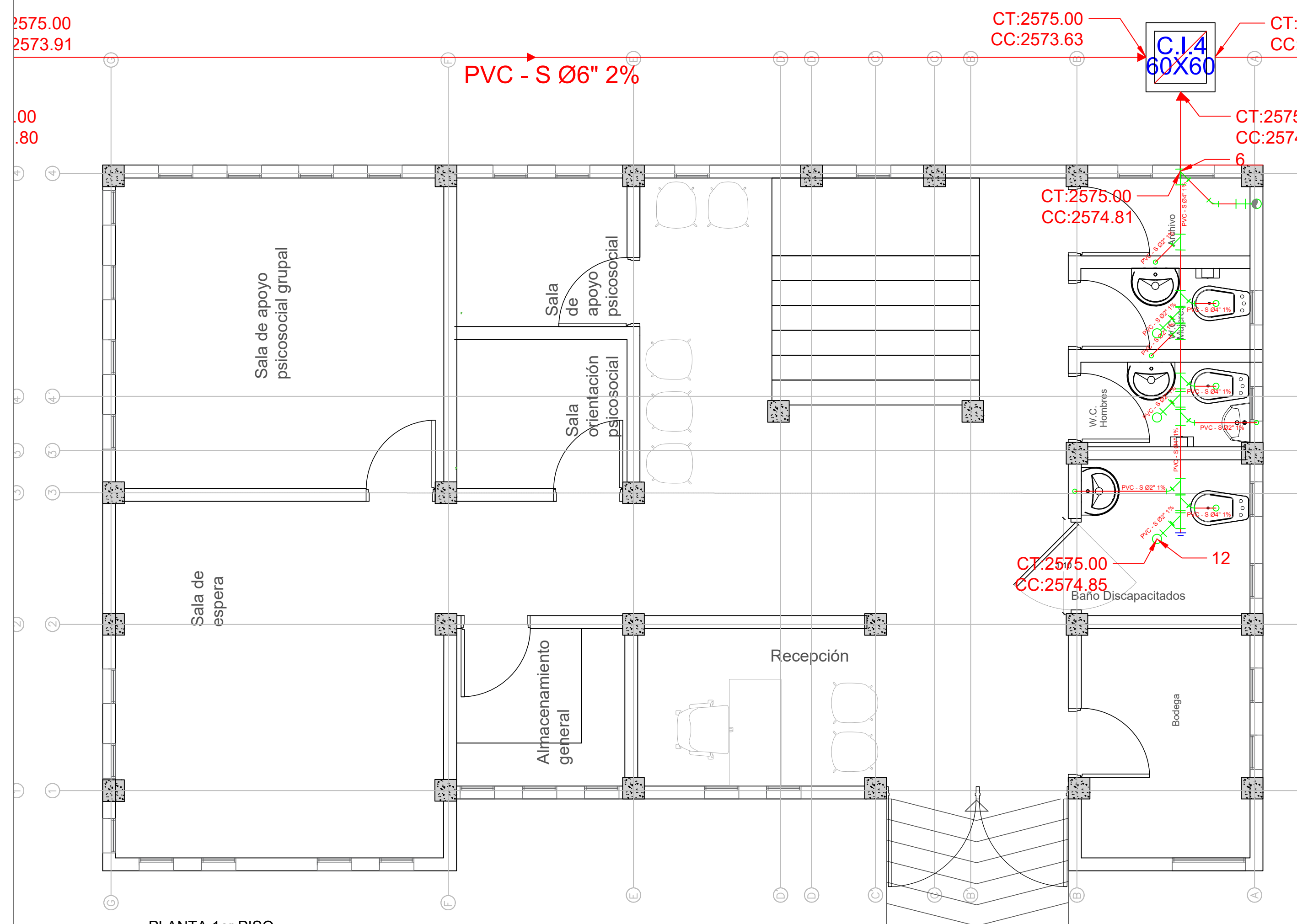
PLANTA 1er PISO Esc. 1:75
