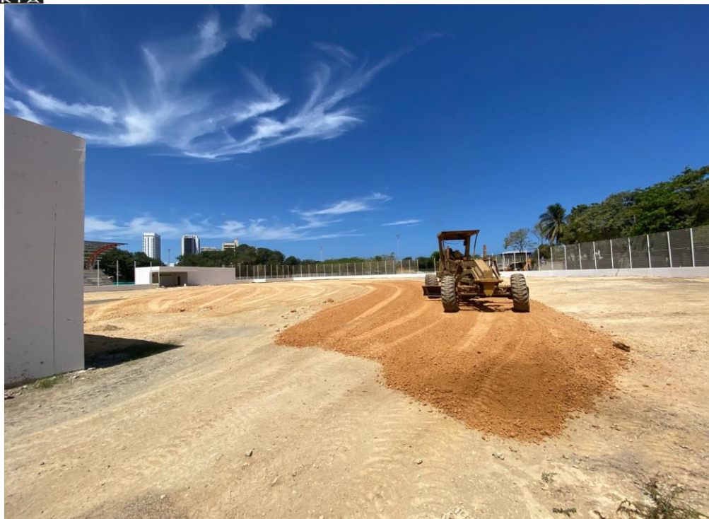
Ilustración 10. Relleno y compactación material seleccionado cancha de softbol.
