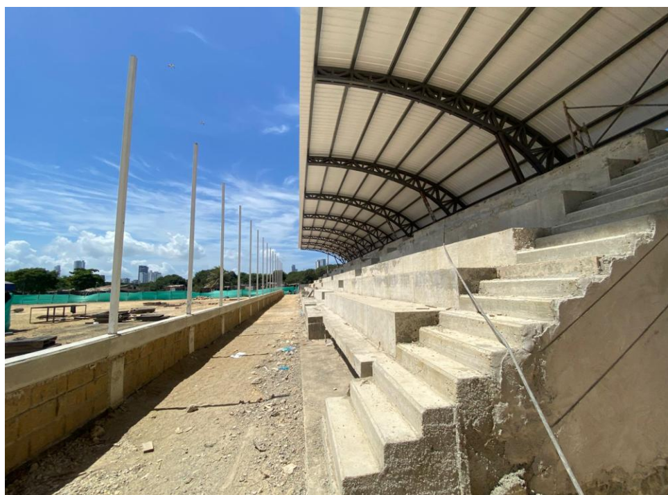
Ilustración 17. Instalación estructura metálica y cubierta graderías de futbol
