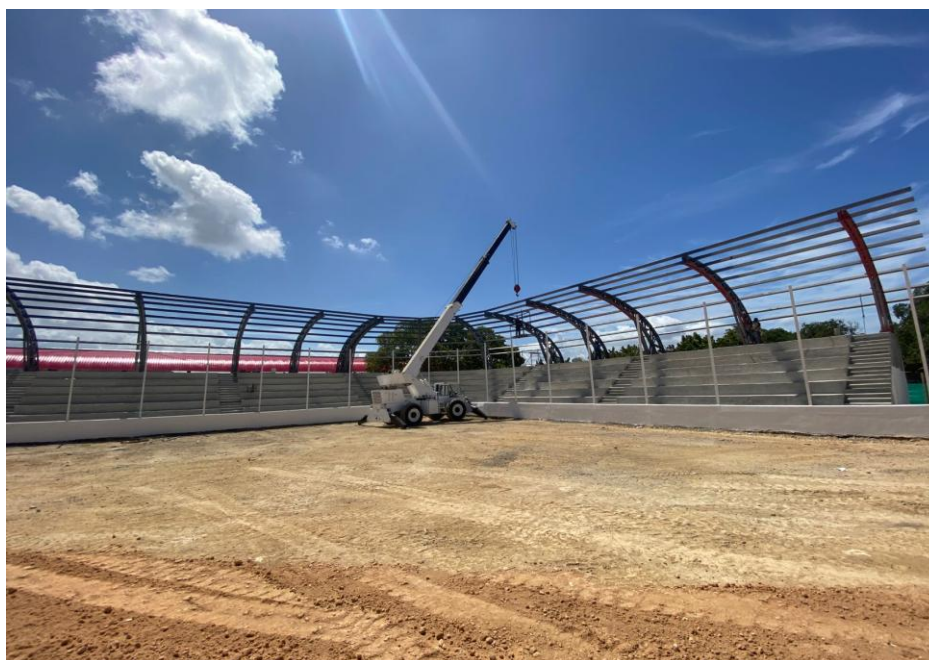
Ilustración 15. Instalación cerchas metálicas para cubierta graderías de softbol
