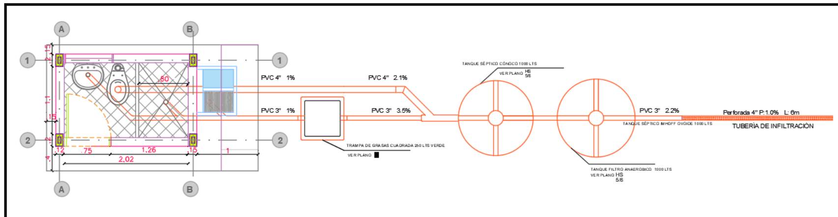
Figura 4. Perfil batería sanitaria, sistema de pretratamiento aguas residuales y campo de filtración
