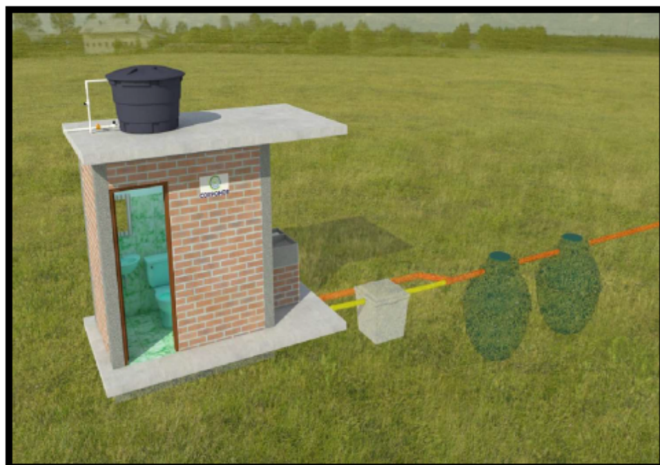
Imagen 3: Isometría general, detalle sistema batería sanitaria
