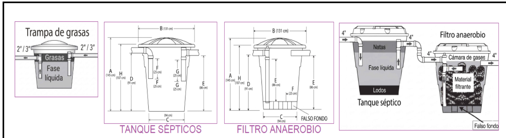
Figura 4. Perfil batería sanitaria, sistema de pretratamiento aguas residuales y campo de filtración
