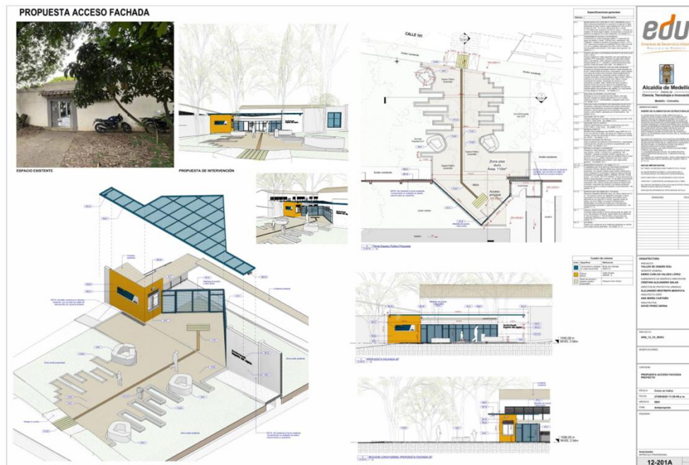
Ilustración 4. Planimetría propuesta de fachada
