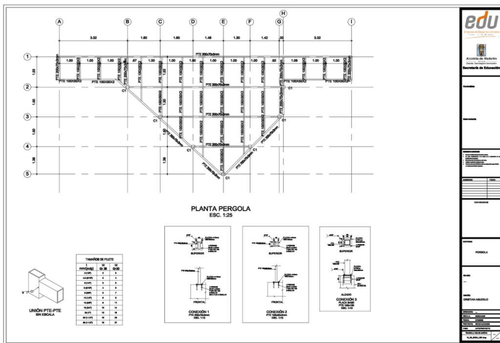
Ilustración 11. Planimetría diseño estructural de pérgola
