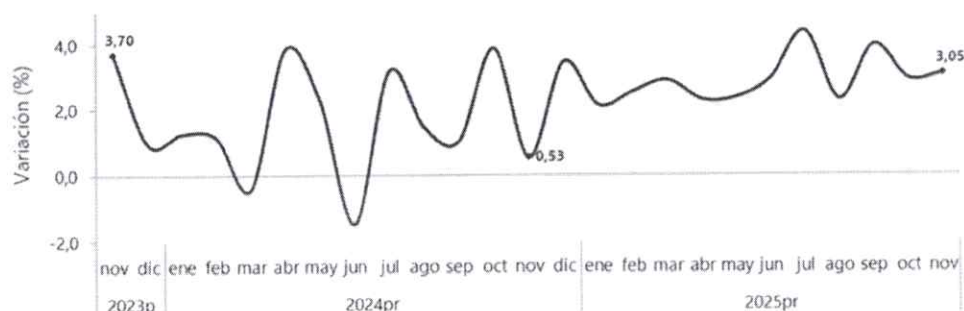
Gráfico 5. Tasa de crecimiento anual del índice del Indicador de Seguimiento a la Economía (ISE) Serie ajustada por efecto estacional y calendario 2023 p - 2025 pr (noviembre)
