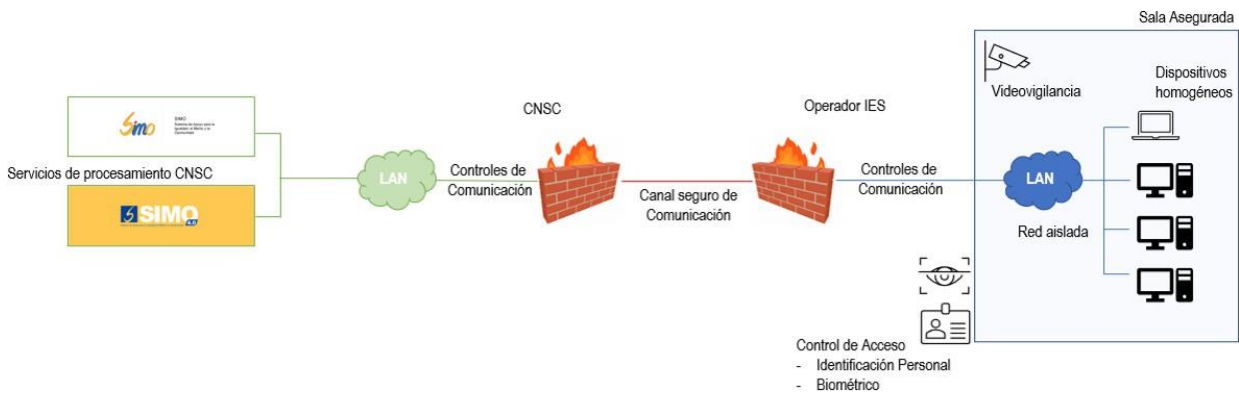
Ilustración 1. Esquema genérico de conexión de salas de trabajo aseguradas que acceden a los servicios de la CNSC
