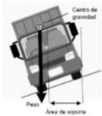
Figura. Área de soporte de un camión.
