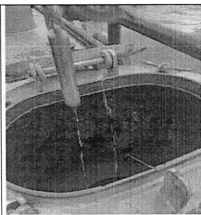
Figura 3: Verificación con crema reveladora de agua.
