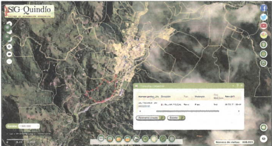
Ilustración 17. Ubicación del predio previsto para la PTAR.
