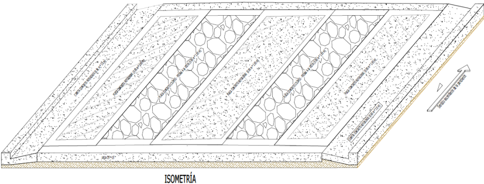
Ilustración 1. Isometría diseño tipo ICCU.
