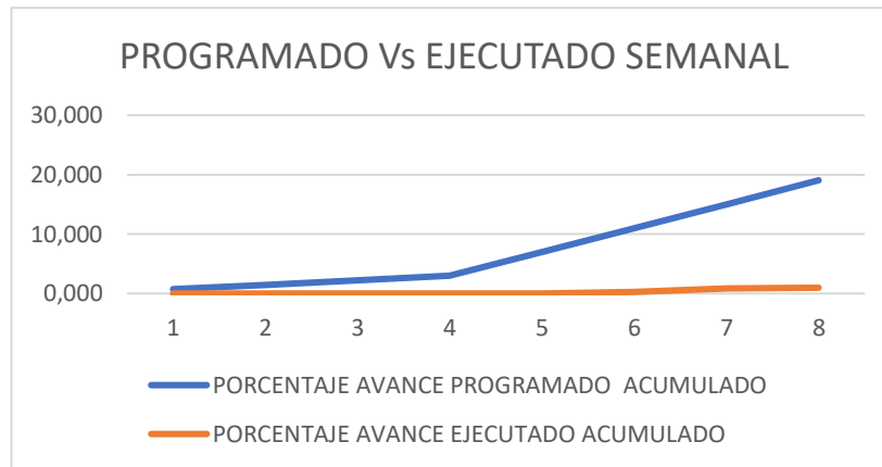
Ilustración 3. Ejecutado acumulado Vs Programado acumulado.
