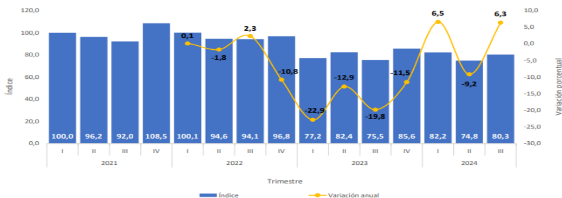
Índice y variación anual de la producción de las carreteras, calles, vías férreas y pistas de aterrizaje, puentes, carreteras elevadas y túneles Total nacional – serie a precios constantes. 2021 (I trimestre) – 2024 (III trimestre Pr )
