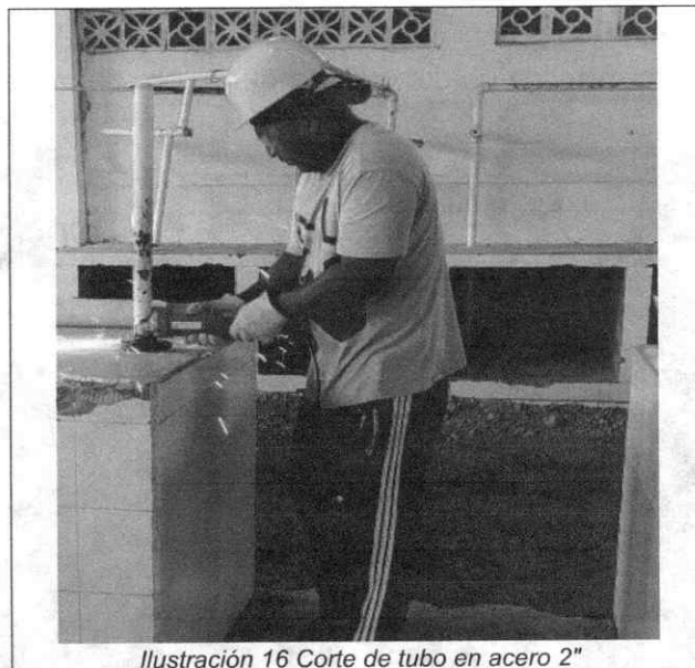
Ilustración 16 Corte de tubo en acero 2"
