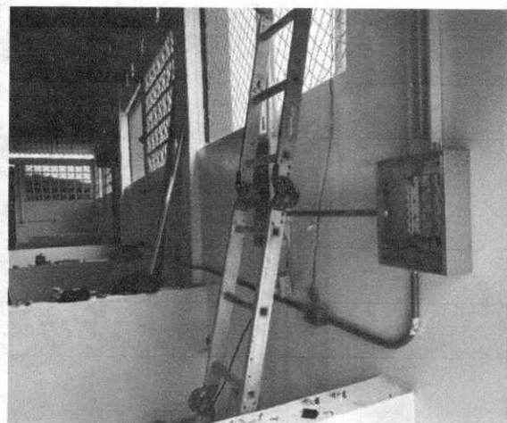
Ilustración 34 Suministro e instalación de tablero trifásico
