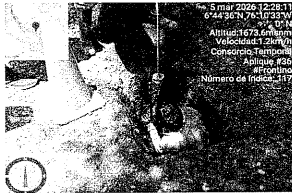
Fotografía 8. Ensayos in situ y toma de muestras en Frontino - Nutibara
