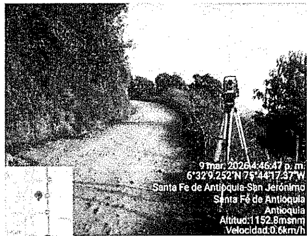
Fotografía 24. Continuación levantamiento topográfico Sopetrán – Horizontes - Belmira
