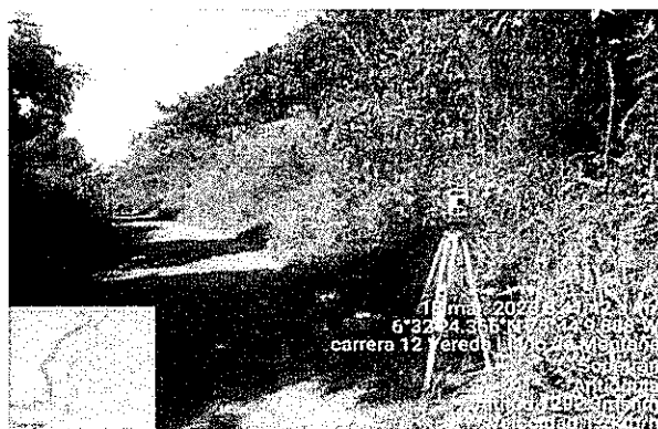
Fotografía 26. Continuación levantamiento topográfico Sopetrán – Horizontes - Belmira
