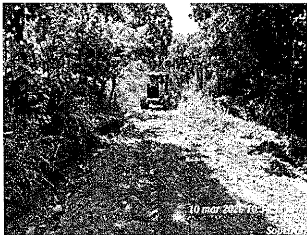
Fotografía 9. Ampliación y conformación del circuito
