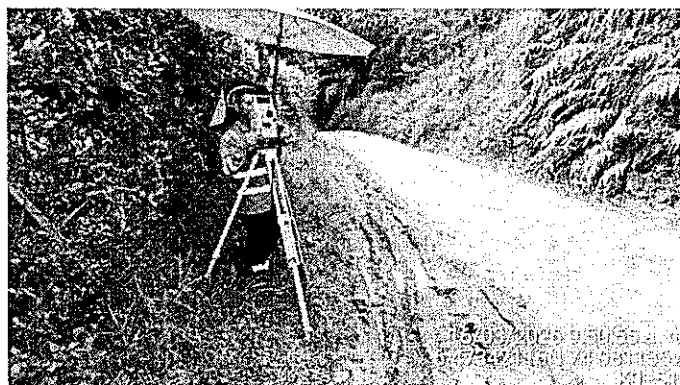
Fotografía 100. Levantamiento topográfico circuito Caramanta – Cristales – San Roque – K9+510
