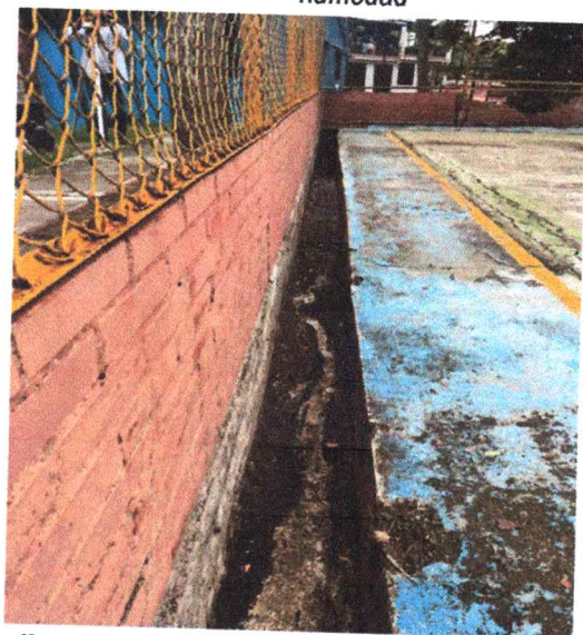
Ilustración 19. Mejoramiento de cuneta para el manejo de aguas lluvias
