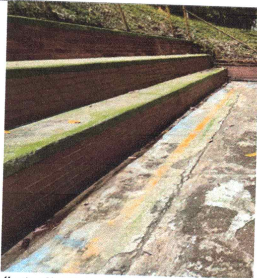
Ilustración 10. Fisuras y Dilataciones en la placa de graderías
