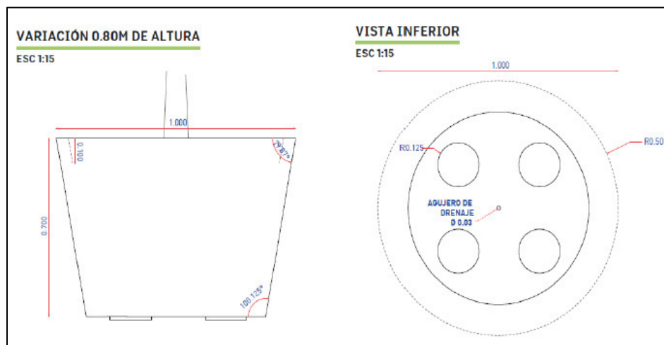
Ilustración 47. Detalle de matera alta
