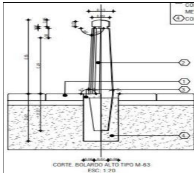
Ilustración 49. Detalle de bolardo M63
