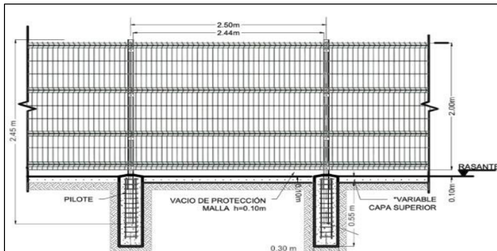
Ilustración 45. Detalle de malla en varilla
