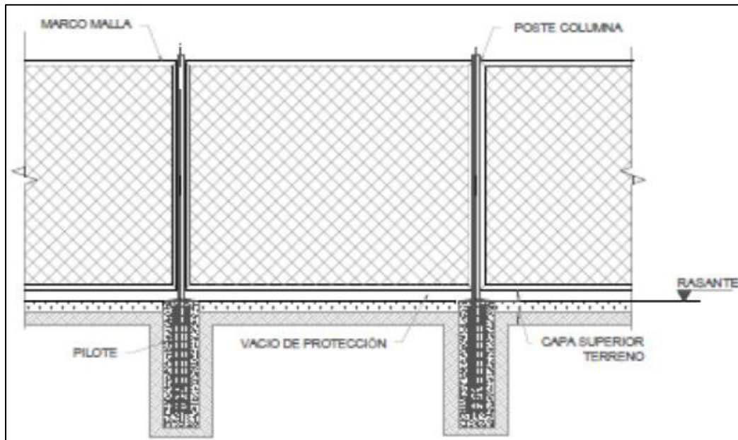
Ilustración 44. Detalle malla eslabonada
