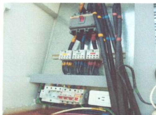
Foto No: 6 Observaciones Particulares: Suministro e Instalación de dps Protección Contra Tensiones Tipo 1+2 Polos / BR 12.5M 4P- MASTIL No.2
