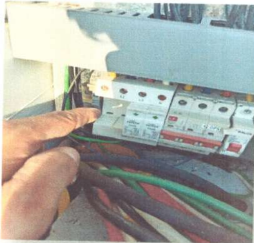
Instalación de DPS Protección Contra Tensiones Tipo 1+2 Polos / BR 12.5M 4P-
