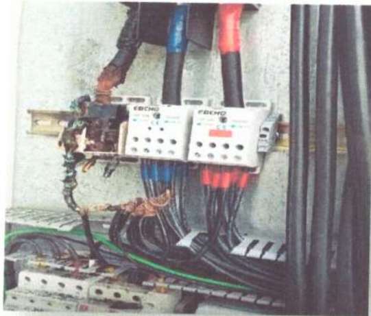
Instalación de DPS Protección Contra Tensiones Tipo 1+2 Polos / BR 12.5M 4P-
