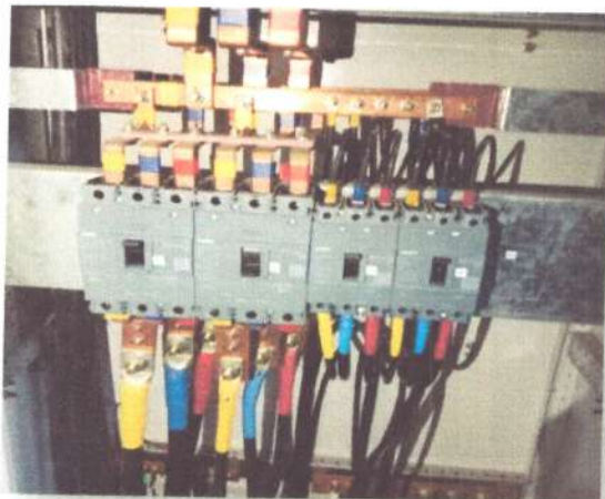
Instalación de Contacto Trifásico 250A 11B25000220 BOBINA 22VAC
