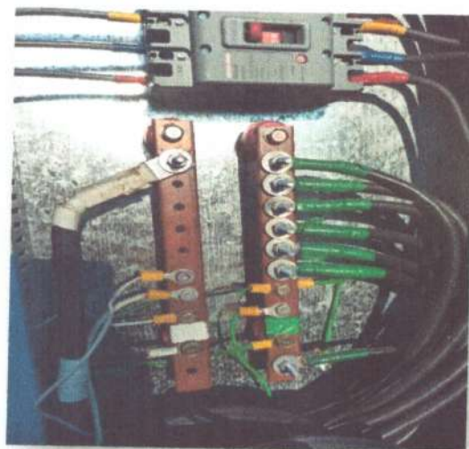
Instalación de Contacto Trifásico 250A 11B25000220 BOBINA 22VAC
