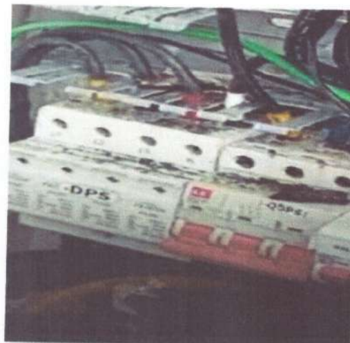
Instalación de DPS Protección Contra Tensiones Tipo 1+2 Polos / BR 12.5M 4P-
