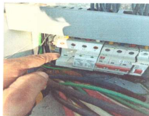
Foto No: 7 Observaciones Particulares: Suministro e Instalación de dps Protección Contra Tensiones Tipo 1+2 Polos / BR 12.5M 4P- MASTIL No.2
