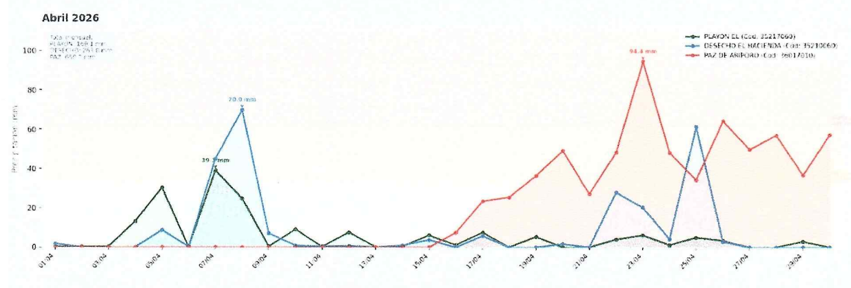
Ilustración 2. Análisis de precipitación diarias por estación IDEAM. Año 2026. Abril. Elaboración propia
