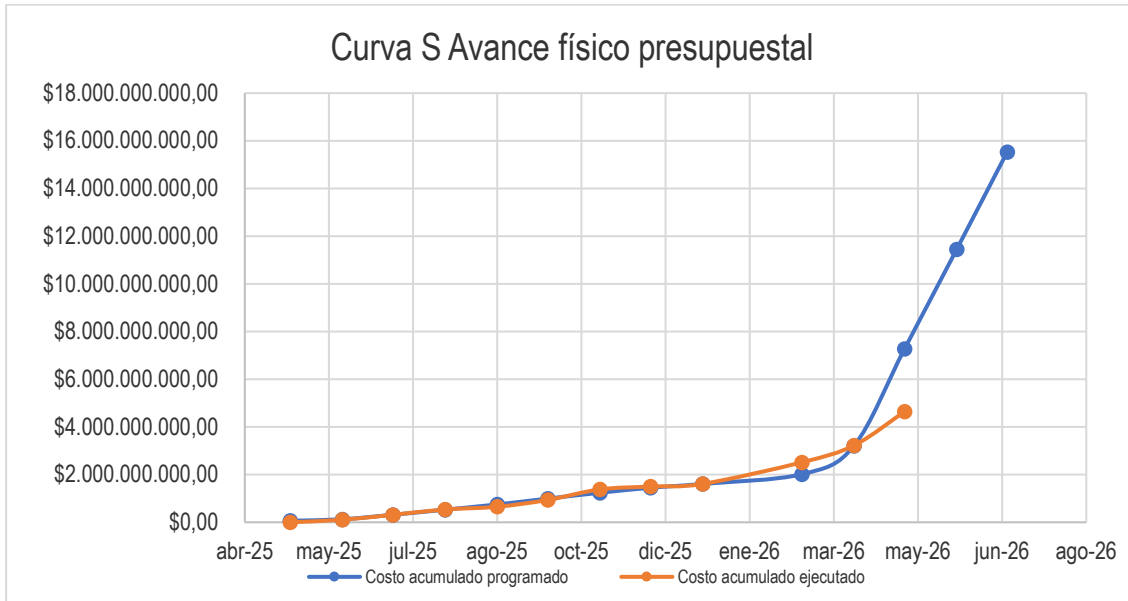
Ilustración 7. Curva S – Avance Físico Presupuestal del presente período Fuente: Elaboración propia.
