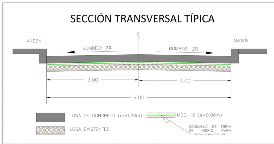
Ilustración 4. Sección de diseño estructura de pavimento
