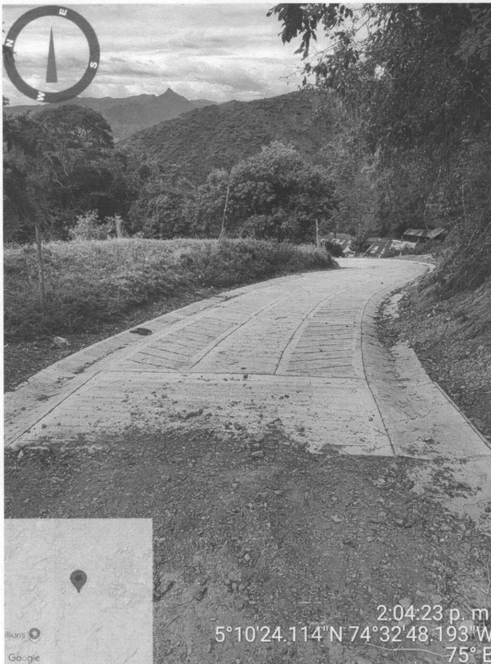
Imagen 7. Placa huella Vda. Barbascales, sector La Escuela.
