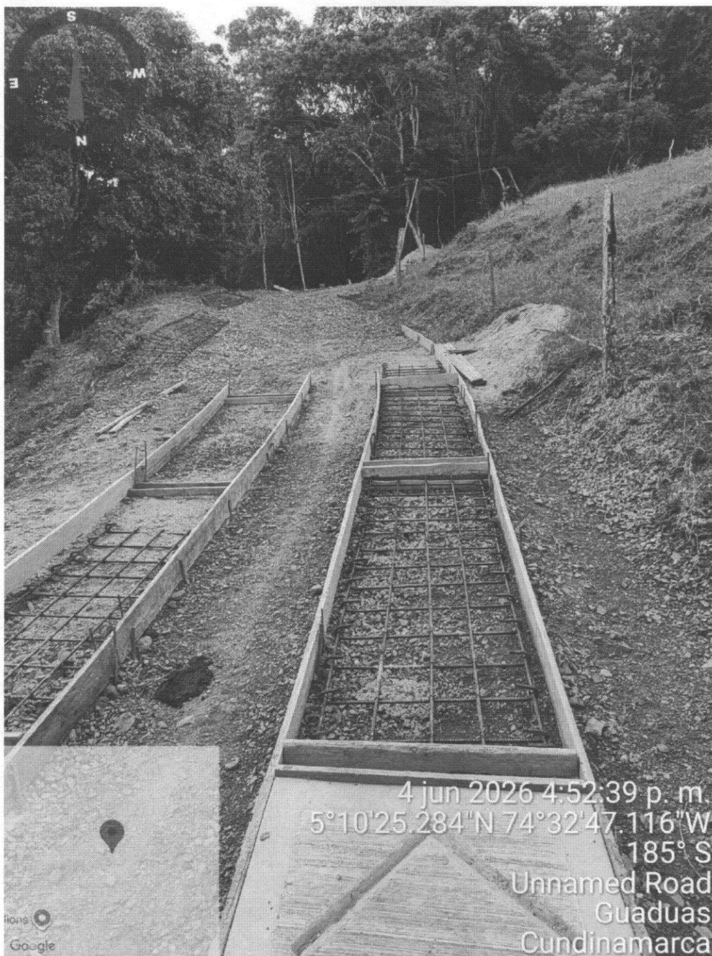
Imagen 12. Placa huella Vda. Barbascales, sector La Escuela.
