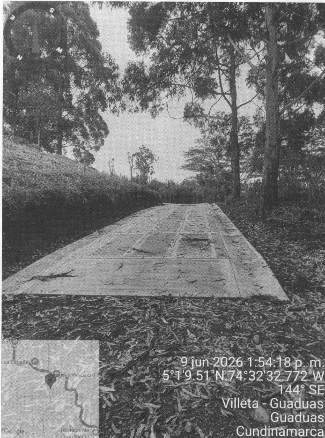
Imagen 17. Placa huella Vda. Balú, sector Casa Vargas.
