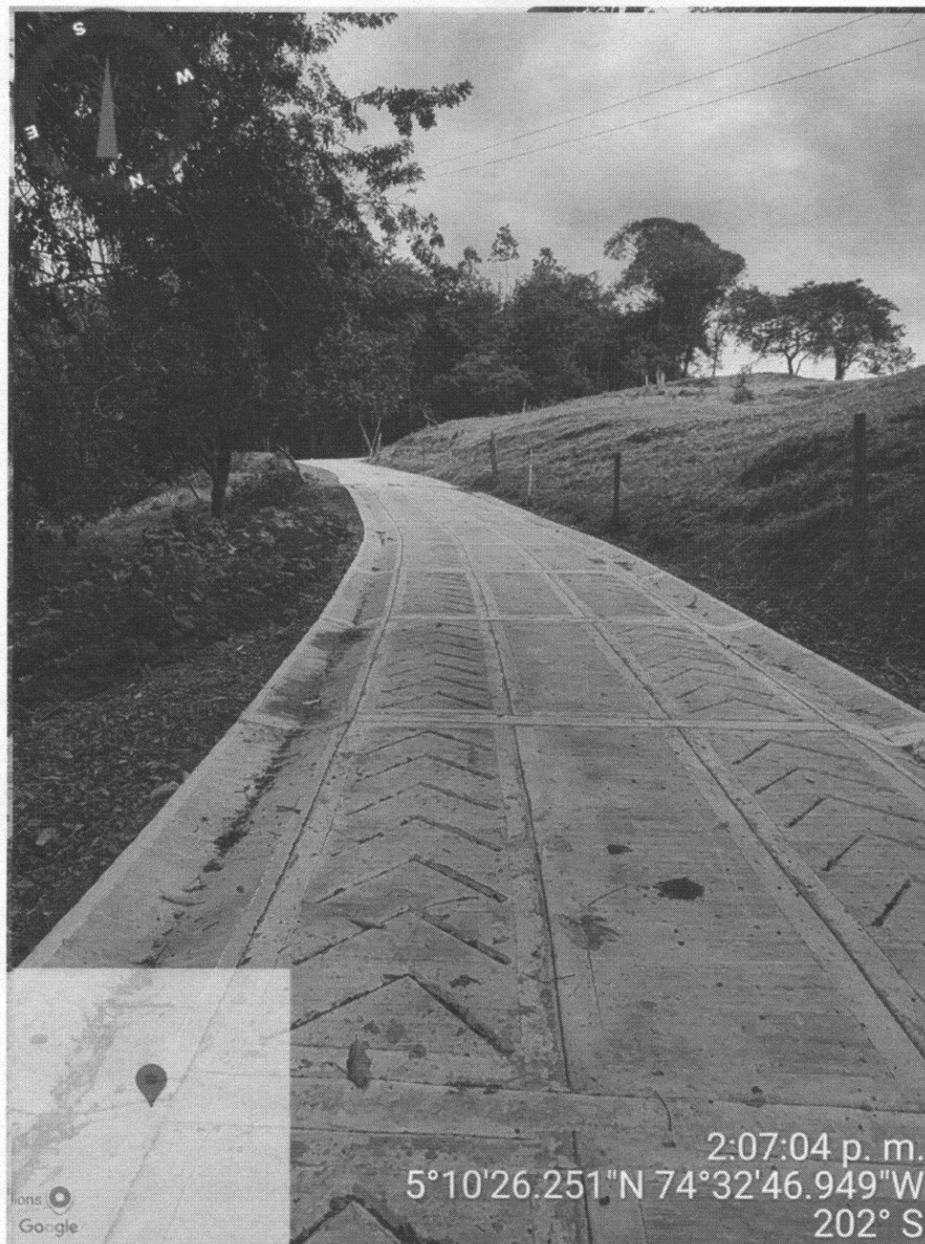
Imagen 6. Placa huella Vda. Barbascales, sector La Escuela.
