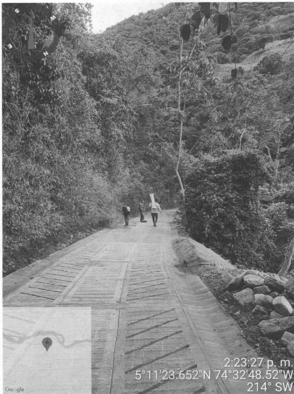
Imagen 4. Placa huella Vda. Barbascales, sector La Zeta.
