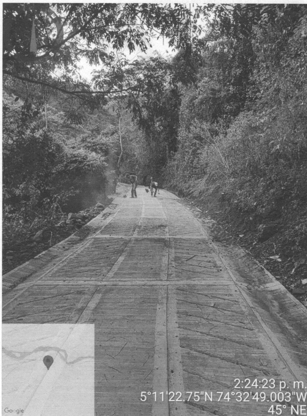
Imagen 1. Placa huella Vda. Barbascales, sector La Zeta.
