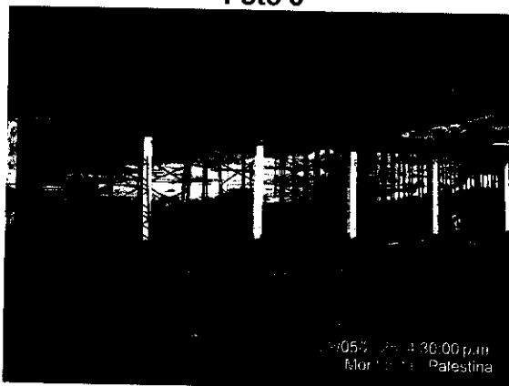
Instalación formaleta metálica Viga canal Eje B
