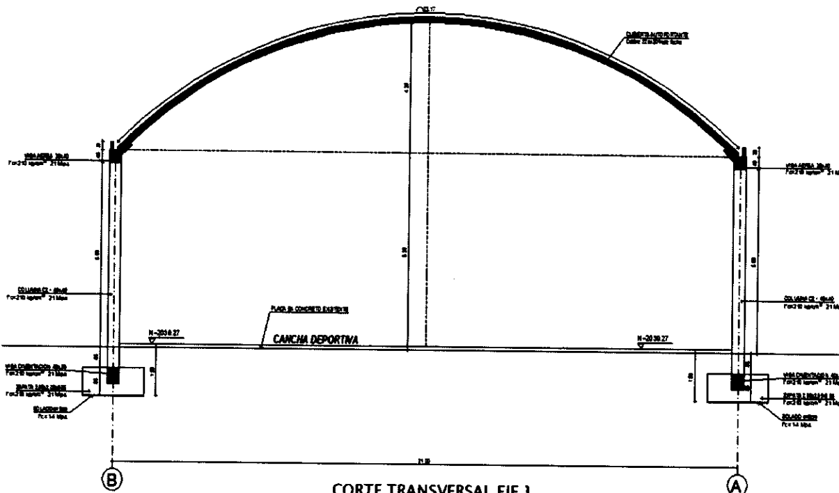
CORTE TRANSVERSAL EJE 1
