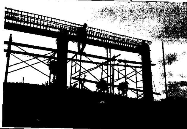
Montaje Acero viga canal eje A
