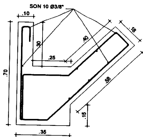
3.05 Plano instalación de manto zetal viga canal.
