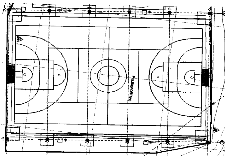
NP 5.07 Plano construcción reposición de Cerramiento perimetral en malla eslabonada hasta, H= 2.5 mt.
