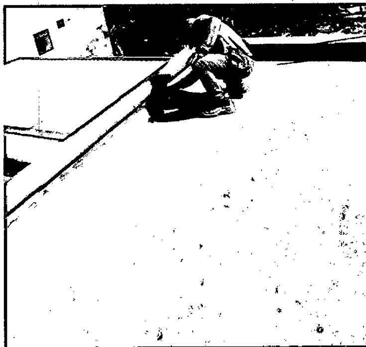
Impermeabilización de losa de cubierta y lagrimales.
