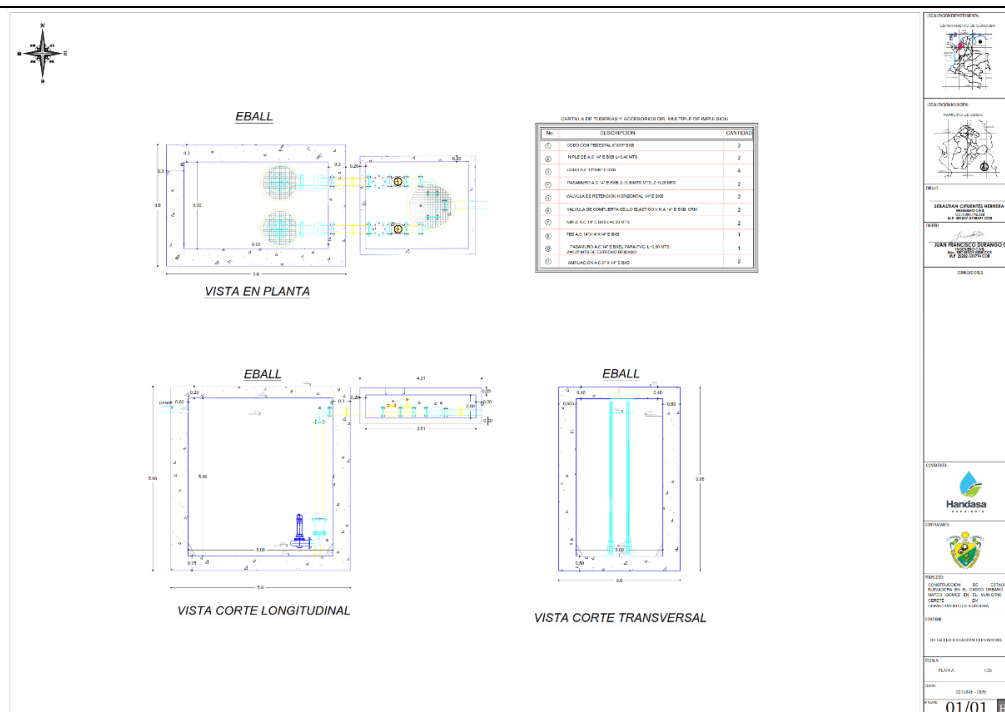
GRAFICO N° 3: PLANOS ESTRUCTURALES
