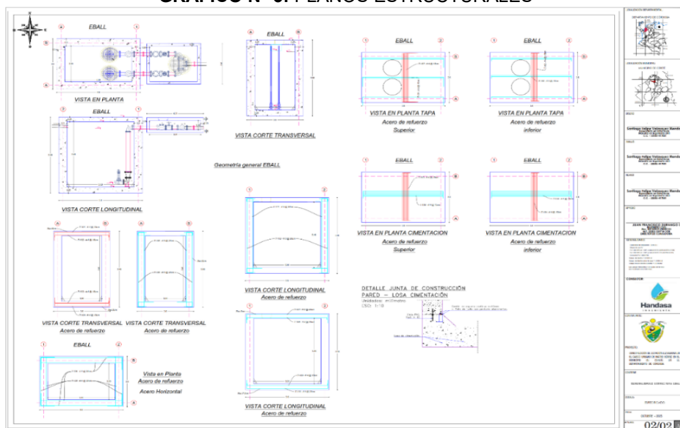
GRAFICO N° 3: PLANOS ESTRUCTURALES
