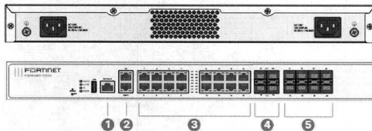
Ilustración 1 Interfaces Firewall
