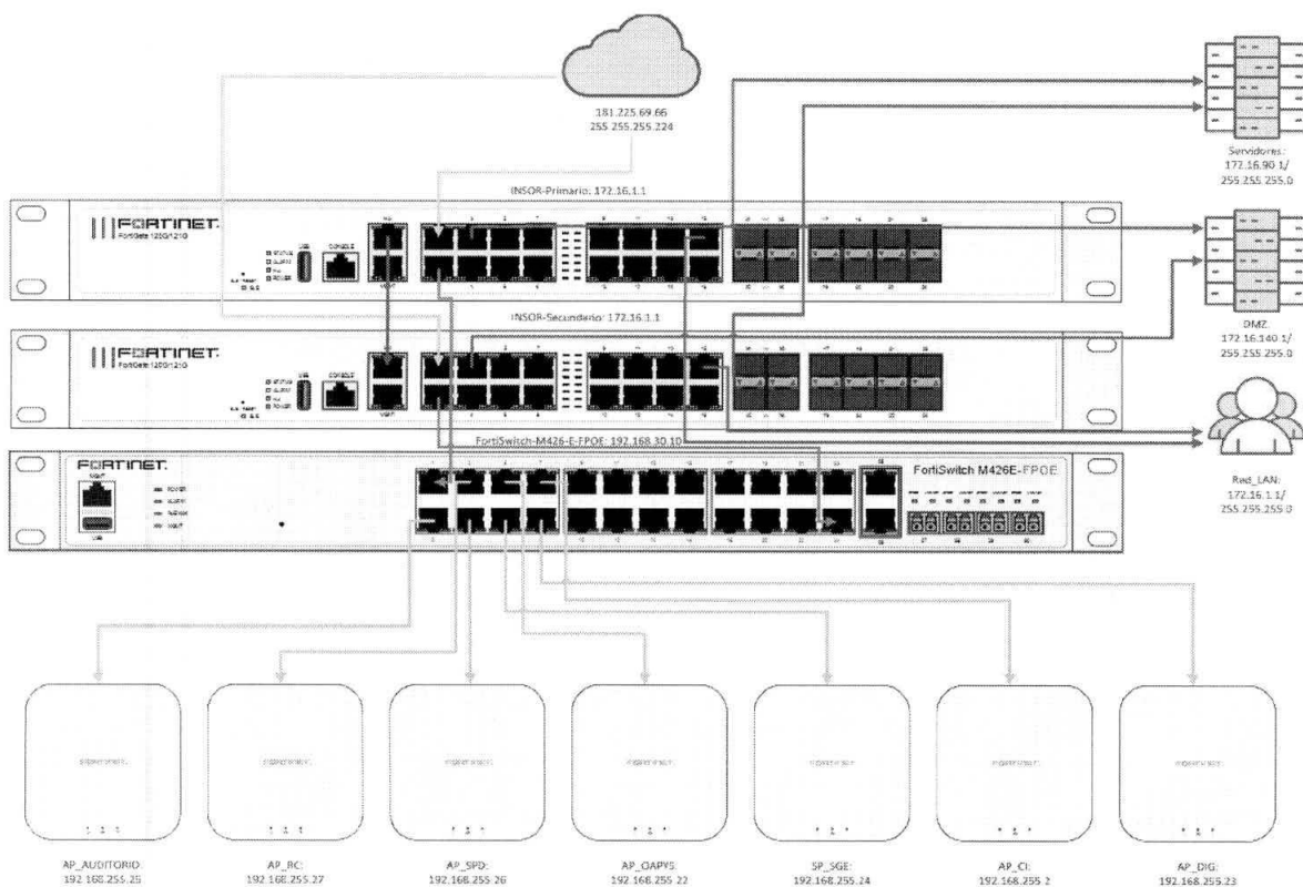
Ilustración 6 Diseño Lógico
